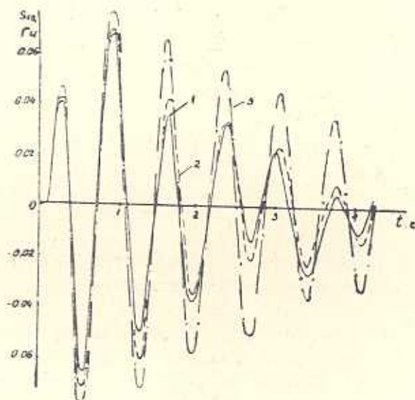
Рис. 2. Зависимость взаимного скольжения s_{13}(t) при возмущении, соответствующем табл. 3. Генераторы представлены: 1 — подробными моделями; 2 — упрощенными моделями с P_\alpha , выбранными по предлагаемому методу; 3 — упрощенными моделями с P_\alpha = 3 о. е.
