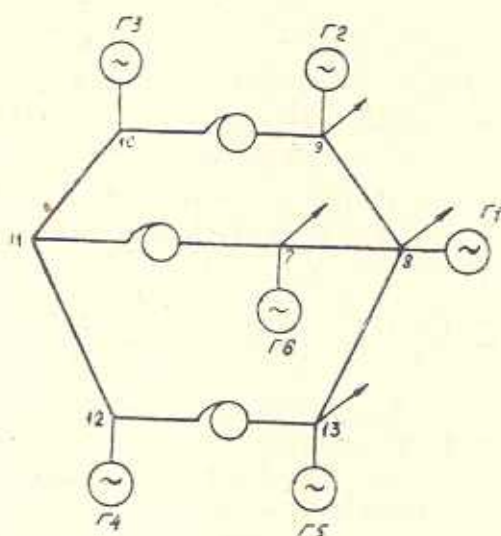
Рис. 1. Схема исследуемой шестимашинной системы.
