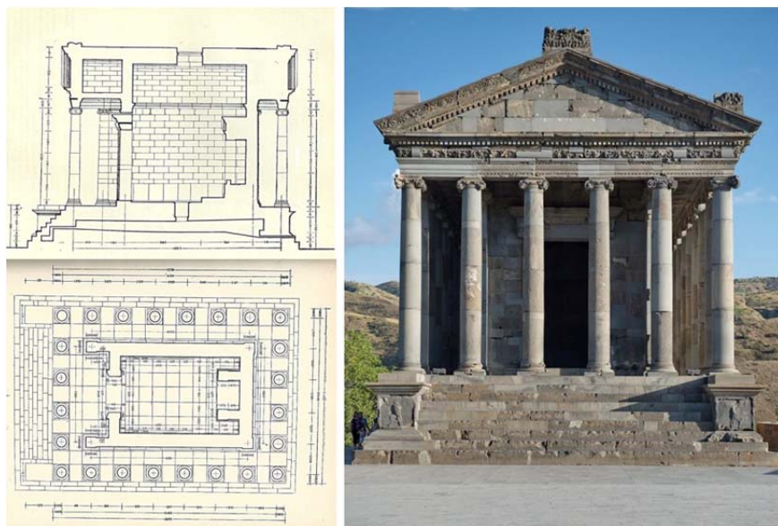
Նկ.16.1- Գաննի հեթանոսական տաճար՝ ճակատ, հատակագիծ, կտրվածք
