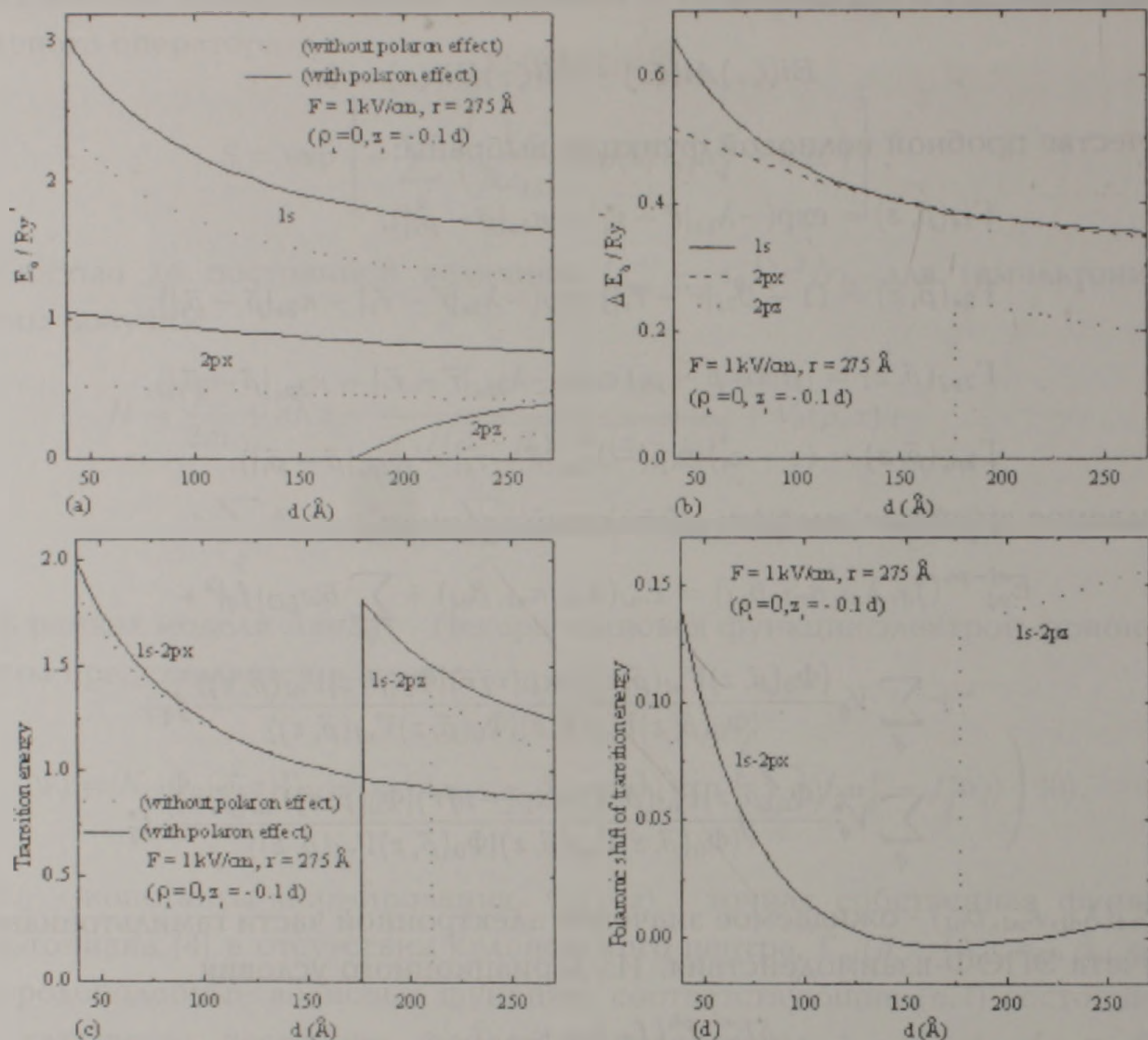
Рис. 1. Зависимость энергии связи примесных состояний 1s , 2p_x , 2p_z (a), поляронные сдвиги этих состояний (b), энергии переходов 1s - 2p_x и 1s - 2p_z (c), а также поляронные сдвиги энергии переходов (d) от длины ЦКТ.
