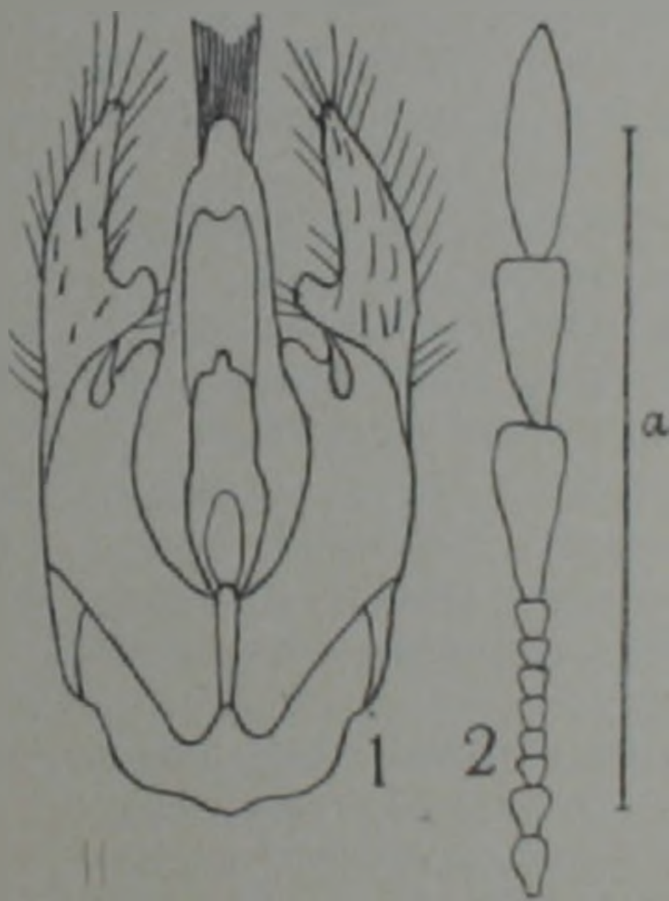
Рис. 2. Anobium ussuriensis Karapetian sp. nov. голотип. 1—пенис вентрально; 2—усик. Масштаб для пениса a=0,5 мм
