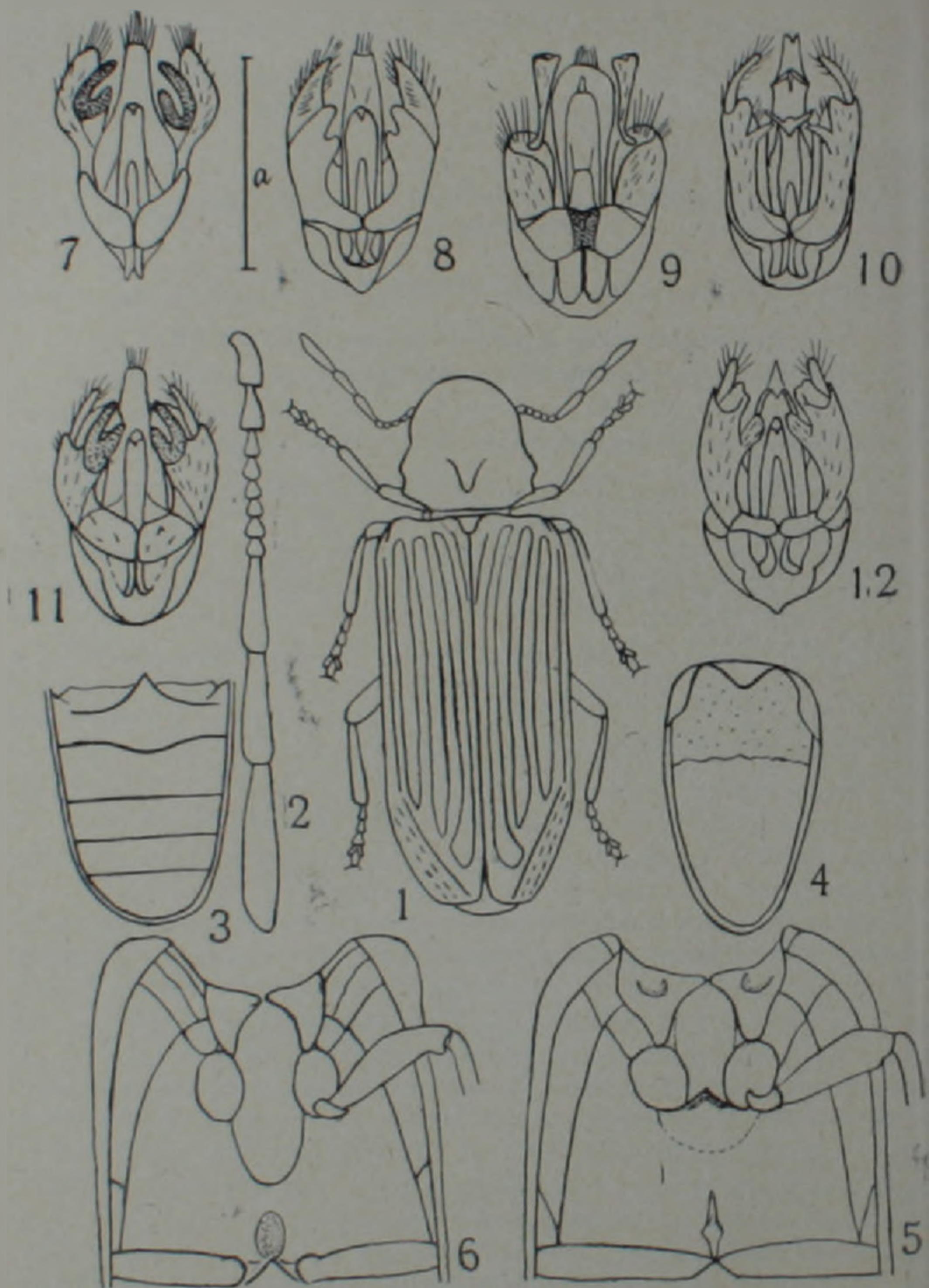
Рис. 1 1—5. Alobium khnzoriani Karapetian голотип: 1—общий вид, 2—усик, 3—брюшко; 4—9-й урит, 5—среднегрудь и заднегрудь, 6—среднегрудь и заднегрудь A. punctatum Deg из Кафана. 7—12. Пенис нейтрально: 7— A. khnzoriani Карар., Гориса, 8— A. costatum Ат. из Алаверди, 9— A. punctatum Deg из Кафана, 10— A. nitidum Herbst из Гориса, 11— A. fulvicorne Sturm из Франции, 12— A. rufipenne Duft. (по Эспаньолу). Масштаб для пенисов: а—0,5 мм
