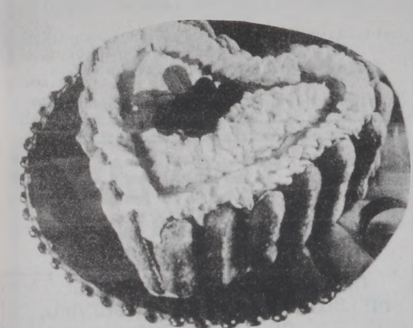
Պատրաստութեան կերպը:
