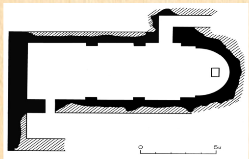
Սուրբ Հովհաննեսի անվան «Վանք» եկեղեցական համալիրի հատակագիծը:
