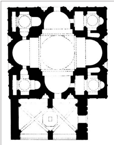
Рис. 7. Церковь Аракелоц (Св. Апостолов) в Ани. План.
