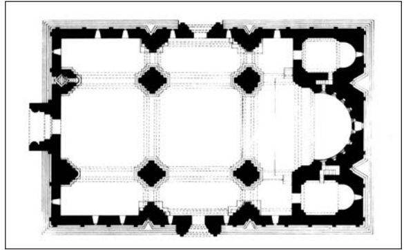
Рис. 2. Кафедральный собор Ани. План.
