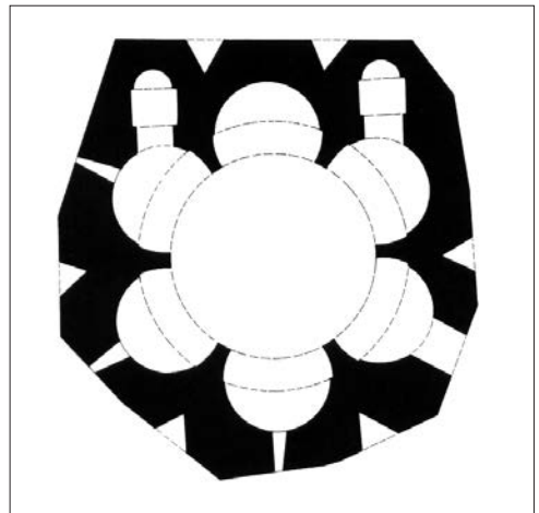
Рис. 8. Церковь Цитадели. План.
