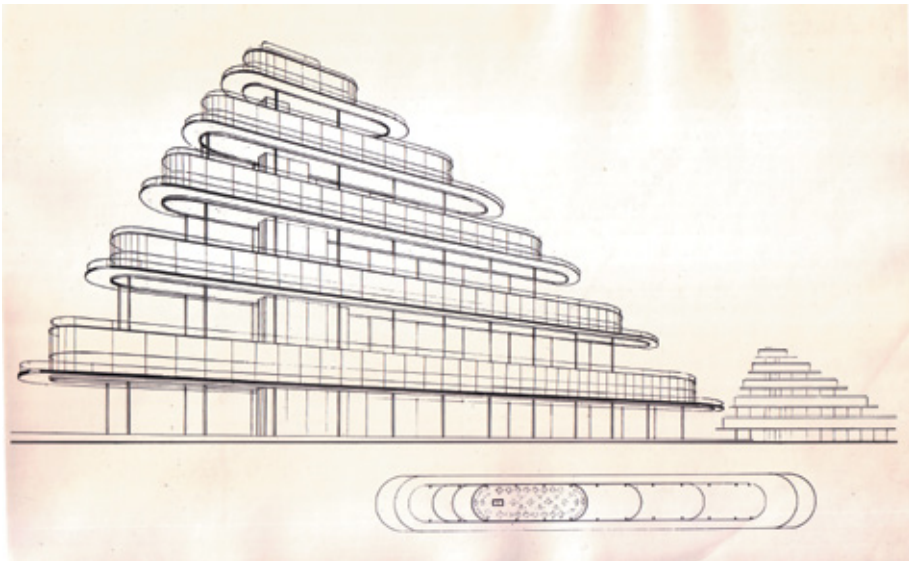
Նկ. 2. Դիպլոմային նախագիծ (Մշակույթի և հանգստի կենտրոնական գրասյգին Մոսկվայում, հյուրանոց, խանութներ, փողավար), 1929: Հեղ.՝ Ճարտարապետ Միքայել Մազմանյան, Մ.Մ-113-3
