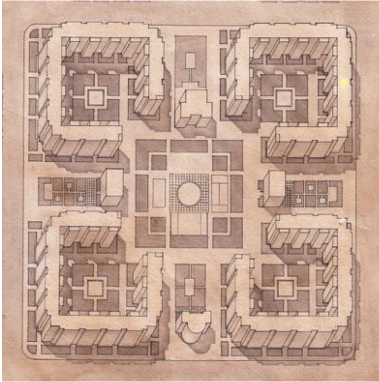
Նկ. 3. Բնակելի թաղամաս սինթետիկ կառուցակի գործարանի բանվորների համար Երևանում, գլխավոր հաղթակազմիծ. (III մաս), 1933: Հեղինակներ՝ Մ. Մազմանյան, Գ. Քոչար, Հ. Մարգարյան, Ս. Սաֆարյան –Մ.Մ-99
