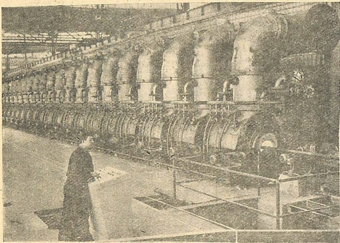
Օստրավայի մետալուրգիական կամբինատի զլոցահատացներից յուրաքանչյուրը կշռում է 5500 տոննա և իր արտադրողականութեամբ համազորը չունի եվրոպայում
