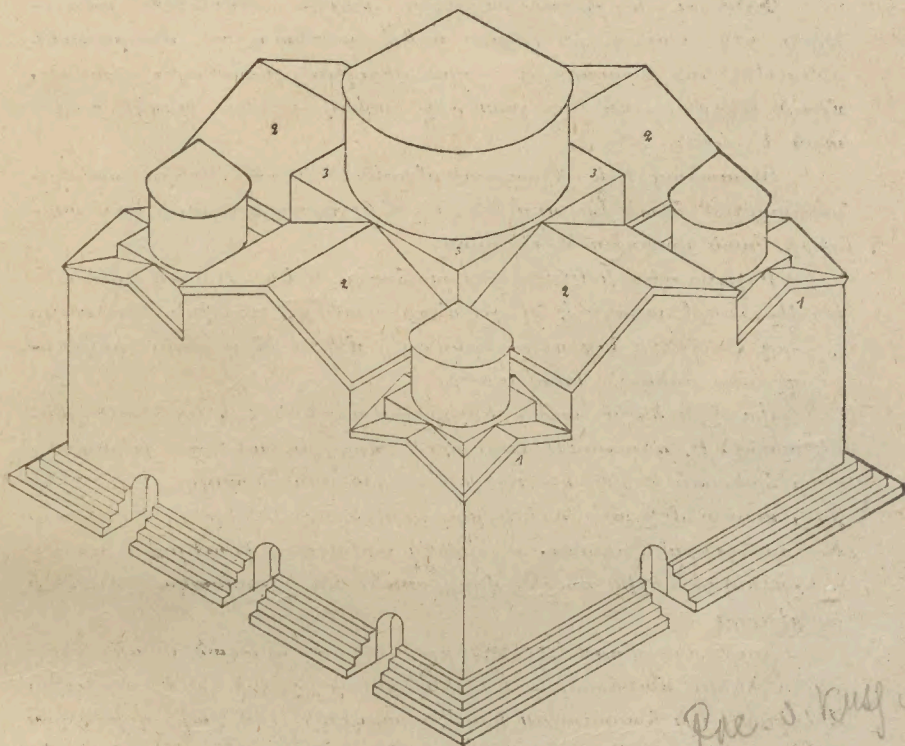
Պատկ. Է. Էջմիածնի տաճարի սկզբնական տեսքը հիւսիս-արեւմուտքից
