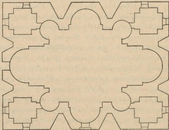
Պատկ. Զ. Ս. Հռիփսիմէի տաճարի մա- կարդակը:
