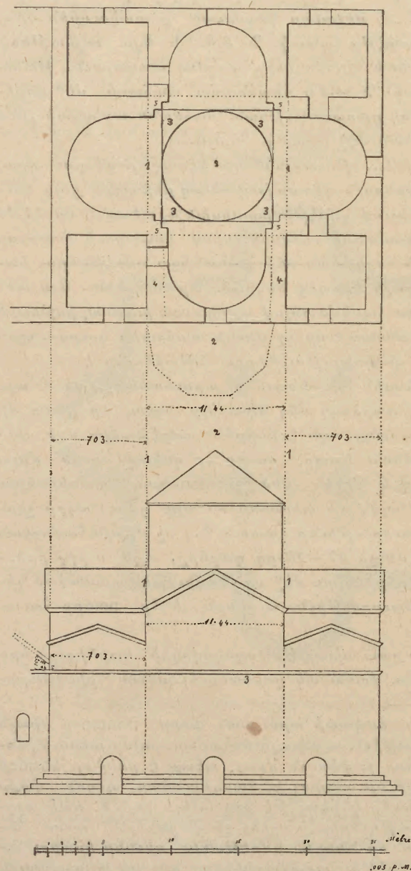
Պատկ. Դ. Էջմիածնի սկզբնական մակարդակը եւ ճակատը՝ հիւսիսից:
