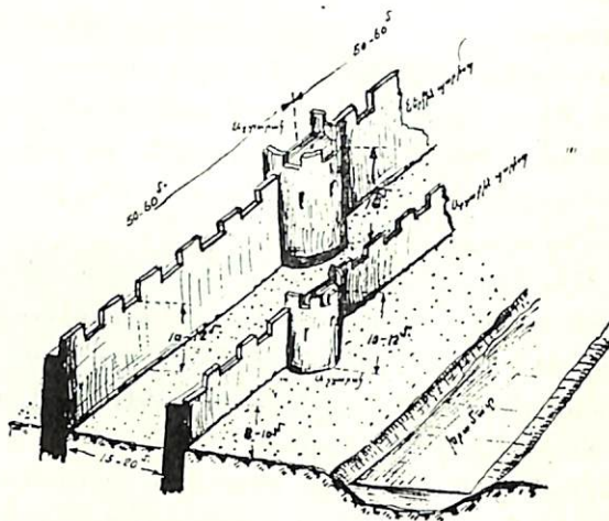
ՊԱՏ. 4. - Հայկական կրկնակ պարիսպներու դասաւորումը.
