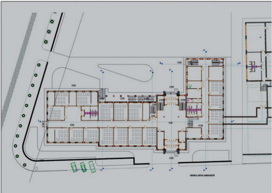
Էօրնեկեան դպրոցի նախագիծը
