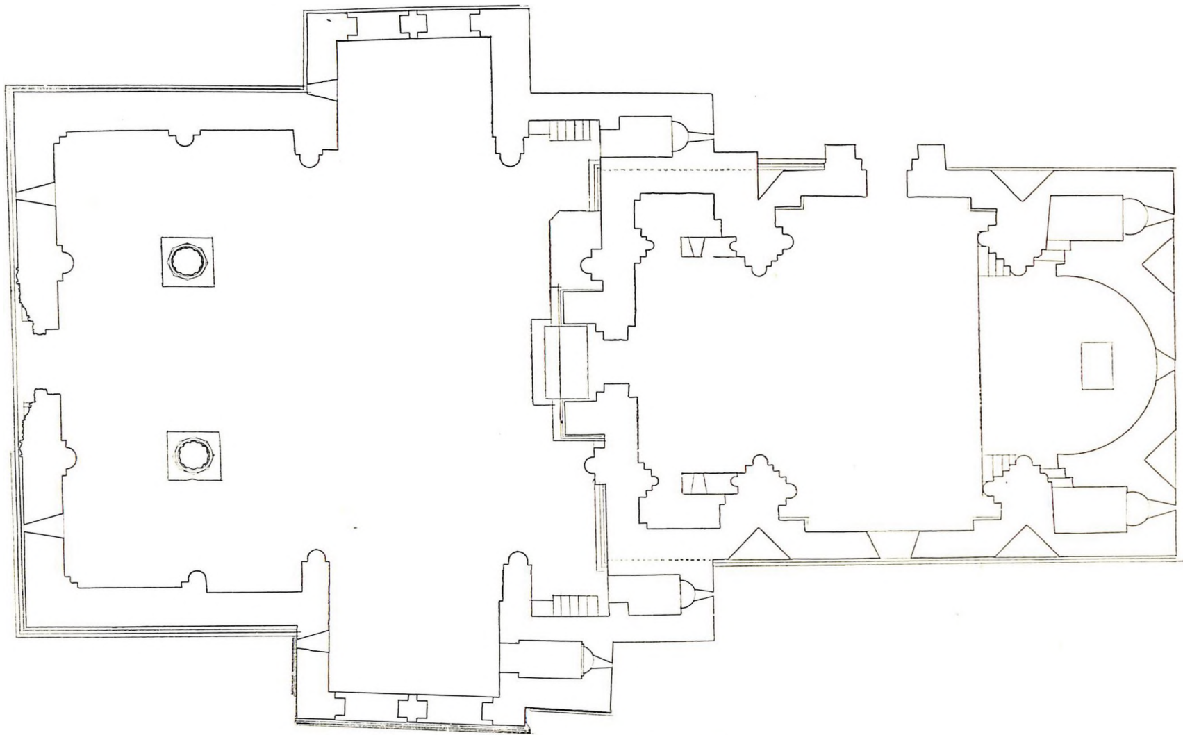
Գլխավոր եկեղեցու և մեծ ժամատան համակարգը
