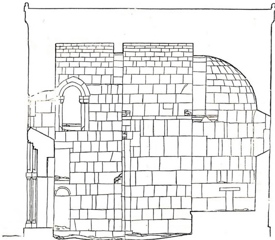
ս. Գրիգոր եկեղեցու երկաթուղիյան կտրվածքը
