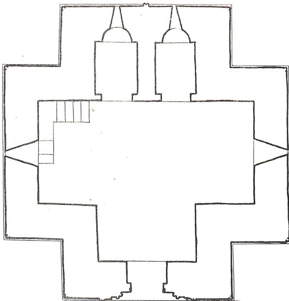
Զանգակատան ստորին հարկի հատակագիր
