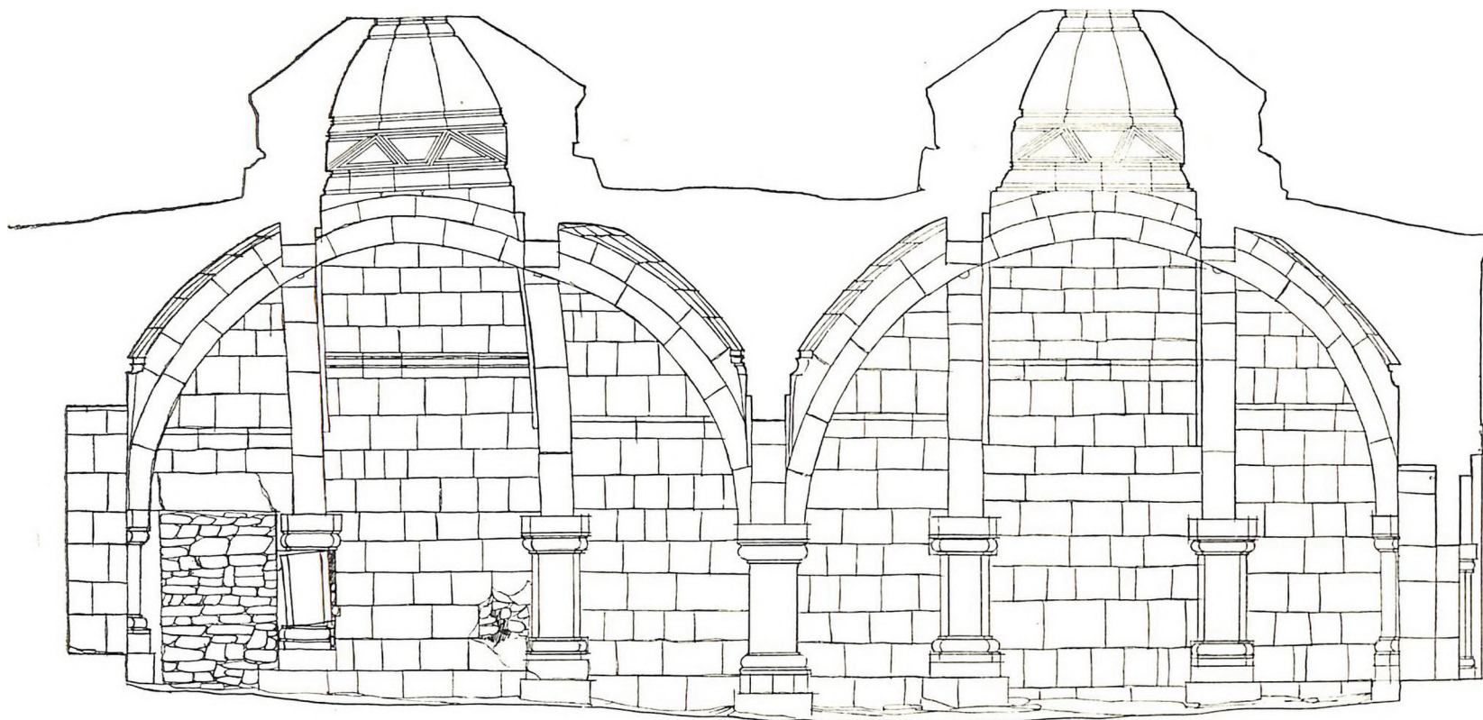
Սեդանատան երկաթյա խճան կտրվածքը
