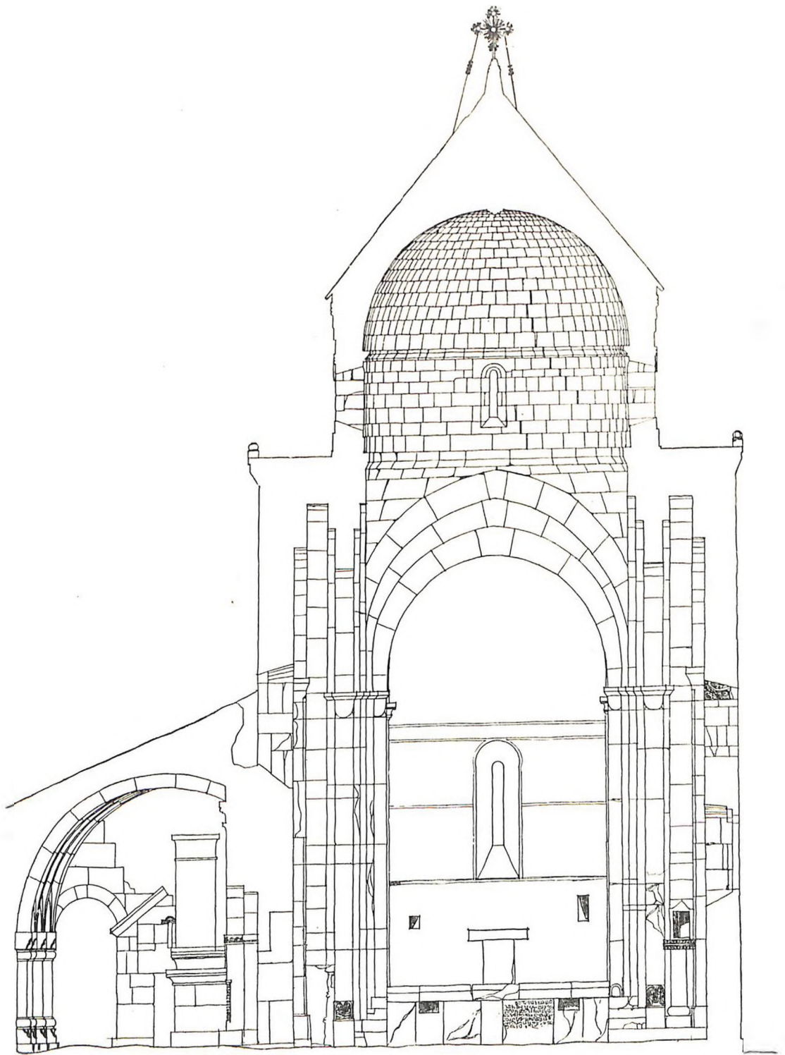
Գլխավոր եկեղեցու և փոքր զավթի լոճների կտրվածքը Տյուսիսից հարավ
