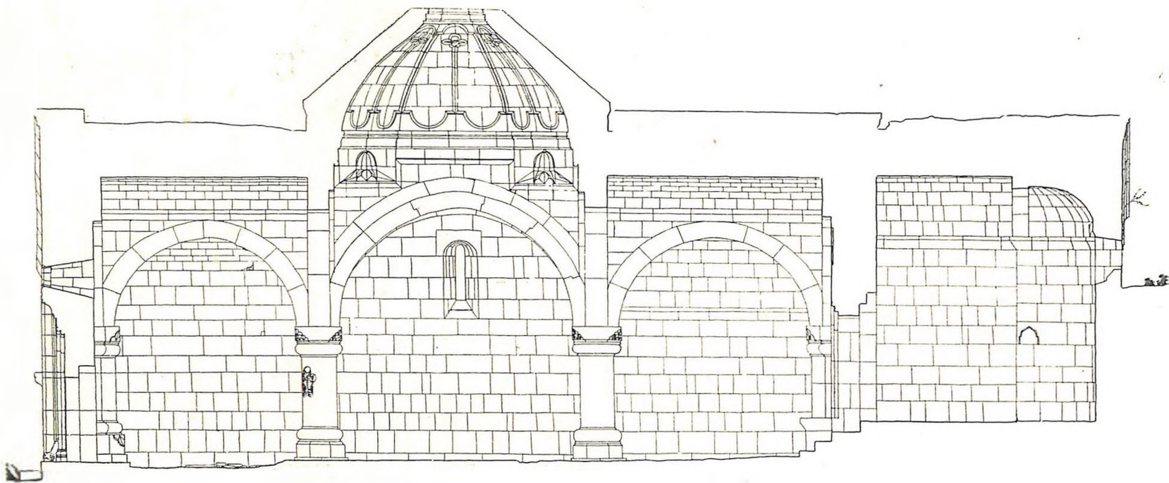
Համապատասխան ժամանակի և նրան կից եկեղեցու, երկարությամբ կտրվածքը
