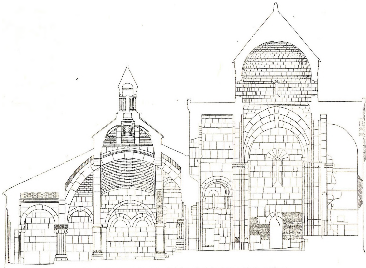
Փլիսափոր եկեղեցու և մեծ ժամատան երկարության կտրվածքը արևելքից արևմուտք
