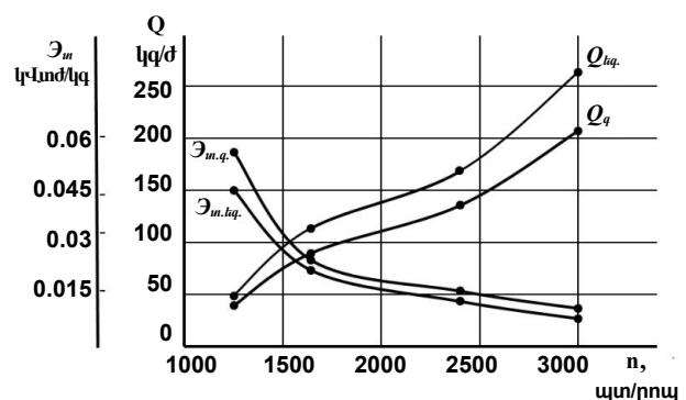
Նկ. 7. Գարու և եգիպտացորենի մանրացման արտադրողականությունը ( Q_{g,q} , Q_{g,iq} ) և էլեկտրաէներգիայի տեսակարար ծախսն ( \mathcal{E}_{m,q} , \mathcal{E}_{m,iq} ) ըստ մանրացնող օրգանի պտուտաթվերի (կազմվել է հեղինակների կողմից):
