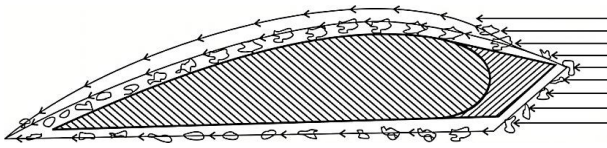
Նկ. 5. Հողամշակ ֆրեզ-մեքենայի դանակի շրջիստելի թևի լայնական հատույթի սխեման (կազմվել է հեղինակների կողմից):
