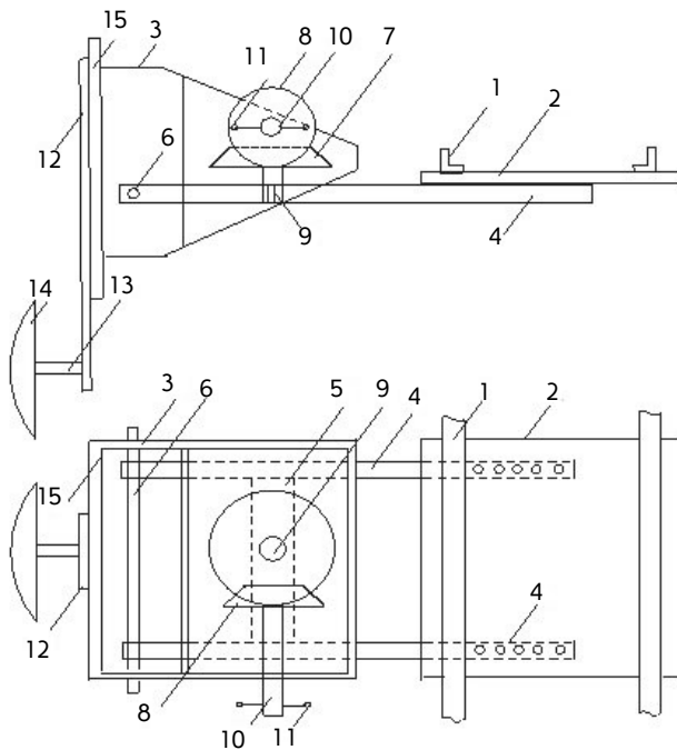
Նկ. 3. Սկավառակի լաբորատոր փորձարկումների ստեղծ. 1 - շրջանակ, 2 - թիթեղ, 3 - իրան, 4 - երկթե եղանիկ, 5 - եղանիկի թևերը միացնող գոտի, 6 - հողակապային սռնի, 7, 8 - ուղղաձիգ և հորիզոնական պտտման առանցքներով ատամնանիվներ, 9 - ուղղաձիգ պտտման առանցքով պարուրակային վերջույթով սռնի, 10 - հորիզոնական պտտման առանցքով ատամնանիվի սռնի, 11 - լծակ, 12 - ուղղաձիգ ձող, 13 - սկավառակ, 14 - սկավառակի սռնի, 15 - իրանի հենապատ (կազմվել է հեղինակի կողմից):
