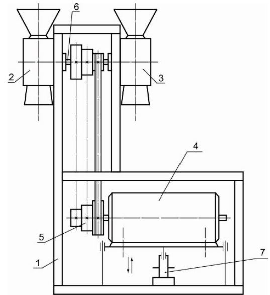
Նկ. 1. Համապիտանի փոքրաչափ կերամանրիչի կառուցվածքային սխեման. 1 - շրջանակ, 2 - հատիկի և հանքային կերատեսակների մուրճային ջարդիչ, 3 - հյութալի և կոպիտ կերատեսակների մանրիչ, 4 - էլեկտրաշարժիչ, 5 - վարիատոր, 6 - լիսեռ, 7 - փոկի ձգվածության կարգավորման մեխանիզմ (կազմվել է հեղինակների կողմից):
