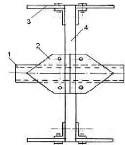
Սկ. 3. Կոպիտ և հյուսիսային կերատեսակների մանրիչի կառուցվածքային սխեման. 1 - լիսեռ, 2, 3 - սեզմենտային դանակներ, 4 - սկավառակ (կազմվել է հեղինակների կողմից):
