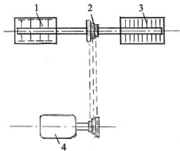
Սկ. 2. Փոքրաչափ համապիտանի կերամանրիչի կառուցվածքային սխեման. 1 - կոպիտ և հյուսիսային կերատեսակների մանրիչ, 2 - պտուտաթվերի կարգավորման վարիատոր, 3 - հատիկային և հանքային կերատեսակների մանրիչ, 4 - էլեկտրաշարժիչ (կազմվել է հեղինակների կողմից):
