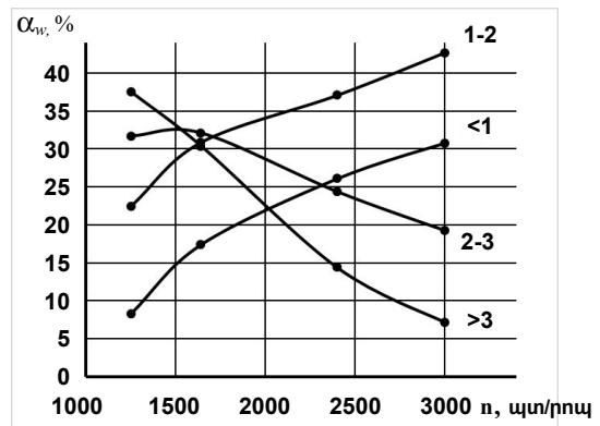
Նկ. 6. Եգիպտացորենի մանրվածքի հատիկաչափական կազմն ( d_{h,eq.} ) ըստ մանրացնող օրգանի պտուտաթվերի ( n_{պ} ) (կազմվել է հեղինակների կողմից):
