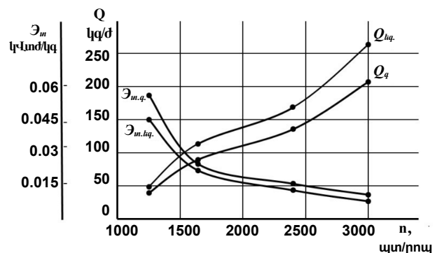
Նկ. 7. Գարու և եգիպտացորենի մանրացման արտադրողականությունը ( Q_{g,q.} , Q_{g,eq.} ) և էլեկտրաէներգիայի տեսակարար ծախսն ( \mathcal{E}_{m,q.} , \mathcal{E}_{m,eq.} ) ըստ մանրացնող օրգանի պտուտաթվերի (կազմվել է հեղինակների կողմից):
