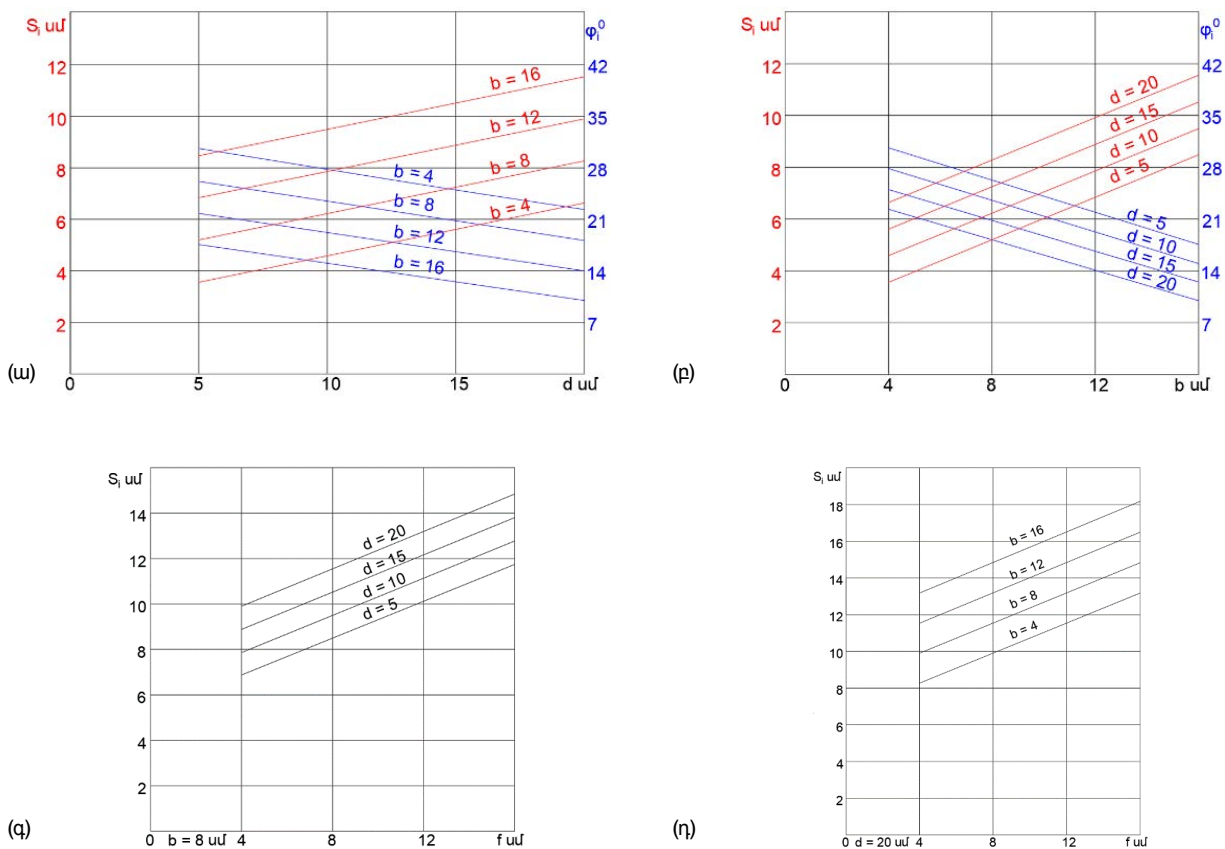
Նկ. 2. Հիդրոգլանի միացի հետընթաց բայի և բանող օրգանի շարժաբևի պտտման անկյան կախվածությունը ծառի տրամագծից (ա), բուսապաշտպան գոտու լայնությունից (բ) և շարքի գծայնությունից ծառաբների շեղվածությունից (գ)՝ m=23 սմ, n=39 սմ, a=8 սմ, c=7,5 սմ, l_w=58 սմ, L_{max}=38 սմ, d_w=32 սմ, e=2 սմ արժեքների համար (կազմվել է հեղինակների կողմից):
