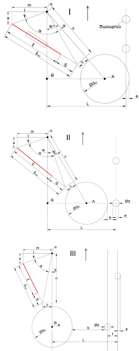
Սկ. 1. Արտաշարժ բանող օրգանի կառավարման համակարգի հիդրոգլանի միացի հետընթաց քայլի և բանող օրգանի շարժաբևեռի պտտման անկյան որոշման հաշվարկային սխեման, երբ բանող օրգանը մշակում է՝ I - միջնային տարածությունը (հիդրոգլանի բաց դիրք), II - մերձնային տարածությունը՝ շրջանցելով շարքի գծայնությամբ դասավորված ծառաբույնը (հիդրոգլանի միջանկյալ դիրք), III - շարքի գծայնությունից շեղված ծառերի մերձնային տարածությունը (կազմվել է հեղինակների կողմից):
