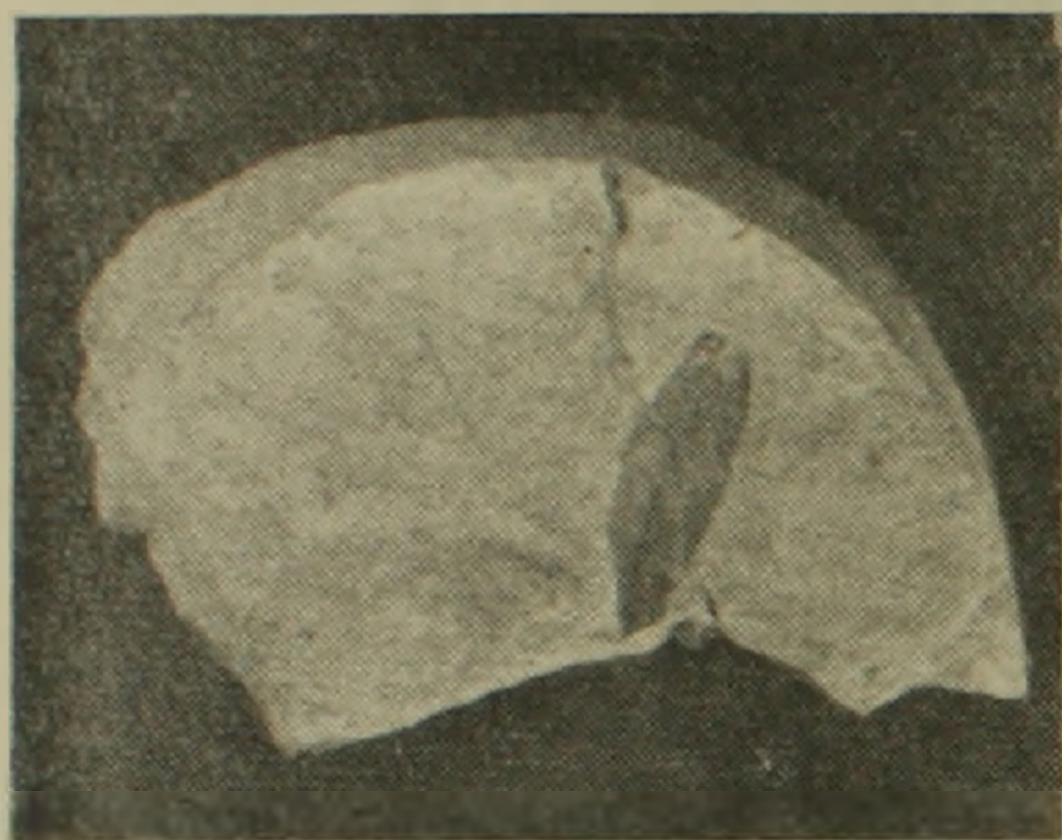
Фиг. 1. Глина. Отпечаток обуглившегося листа. Натур. величина
