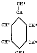
Մէթիլօիլօէկզան Méthylcyclohexane
