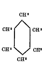
Միջլօէկզան
