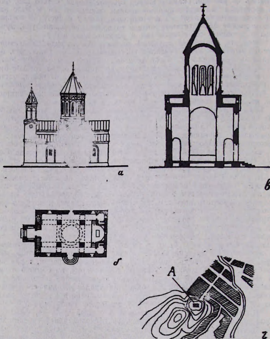
Рис. 2. «Проект армяно-григорианской церкви, во имя воинства св. Полководца Вартана, предполагаемой к постройке в городе Ахалцах», утвержденный исправляющим должность наместника Кавказского, генералом-адъютантом (подпись неразборчива) 31 декабря 1861 года. «а южный фасад; б) план; в) разрез; г) план части города Ахалцыха с обозначением места под литерою А, на коем предполагается постройка церкви по сему проекту». Перерисовано с оригинала, хранящегося в ЦГИА АрмССР, ф. 53, оп. 1, д. 125, л. 5б.
