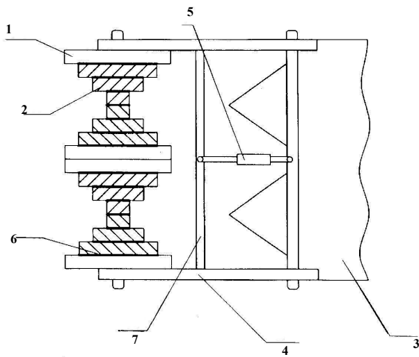
Նկ. 1. Կոշտամանրիչ-փոխակրիչի սկզբունքային սխեման. 1 - ռոտոր, 2 - դանակ, 3 - կարտոֆիլահան մեքենա, 4 - հողակապով լծակ, 5 - կարգավորիչ հարմարանք, 6 - օդագոտի, 7 - հորիզոնական ձող (կազմվել է հեղինակների կողմից):
