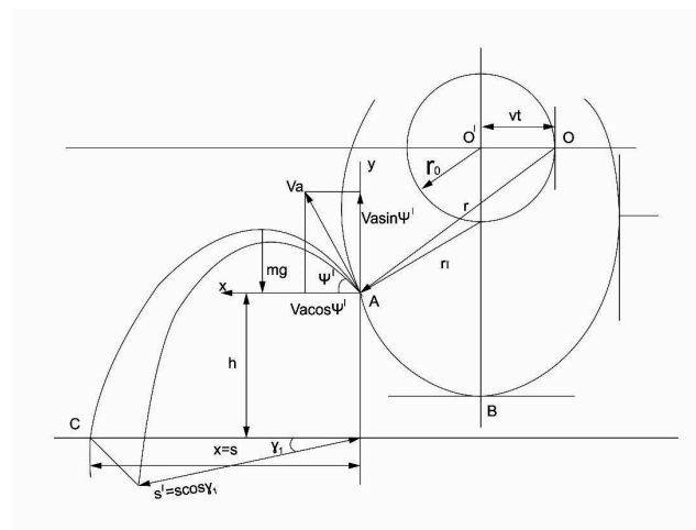
Նկ. 2. Հողային տաշեղի թռիչքի հետազոտության հաշվարկային սխեման ( կազմվել է հեղինակների կողմից ):
