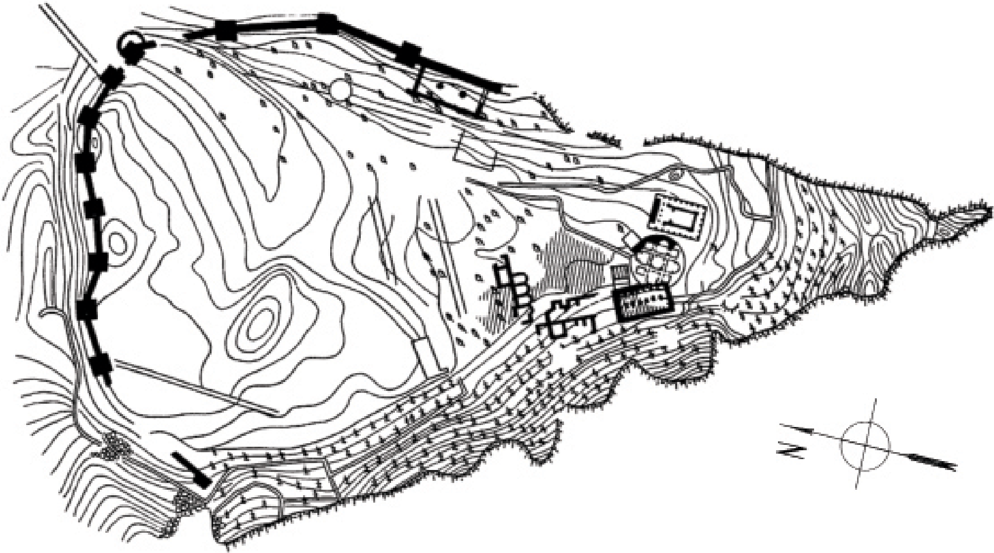
Գառնի ամրոցի ընդհանուր հատակագիծը պարիսպներով և արքունական կառույցների հատվածը
