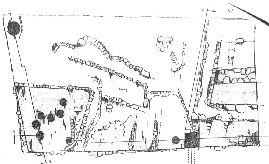
Բջնի ամրոցի ստորին հարթակի պեղված տարածքի հատակագծից՝ ըստ 2003 և 2004 թթ. պեղումների
