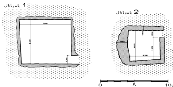
Գծ. 2. Զուլյգ սենյակների սխեմատիկ չափազերություն (չափազեր.՝ Ա. Հախվերդյանի):
