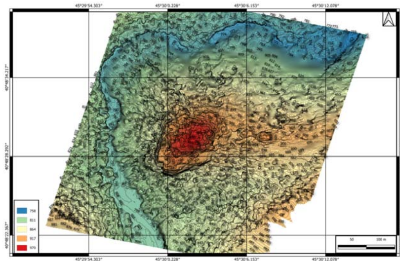
Նկ. 2. Ամրոցի տեղագրական հանույթ (կառ.՝ Լ. Մկրտչյան):
