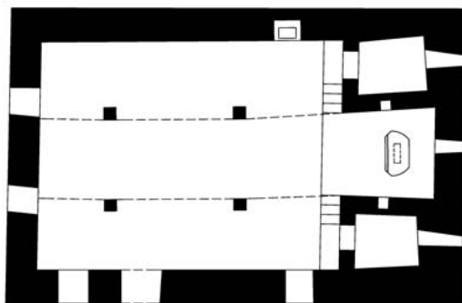
Սր. Կարապետ եկեղեցու հատակագիծը (չափ.՝ Ա. Հակոբ- յանի, 2014 թ.)
