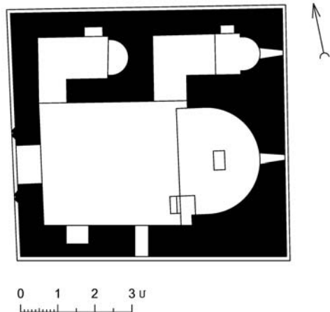
Մր. Պողոս-Պետրոս վանքի ներքին եկեղեցու հատակագիծը (չափ.՝ Ա. Հակոբյանի, 2014 թ.)
