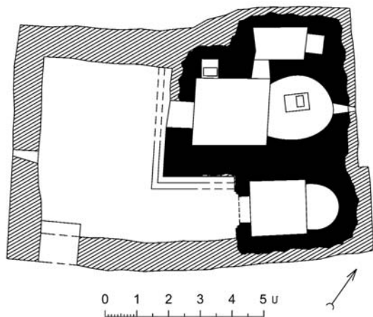
Թուխ մանուկ վանքի հատակագիծը (չափ.՝ Ա. Հակոբյանի, 2018 թ.)
