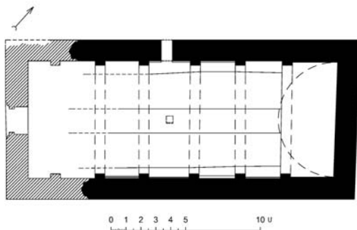
Իջևանատան հատակագիծը (չափ.՝ Ա. Հակոբյանի, 2018 թ.)
