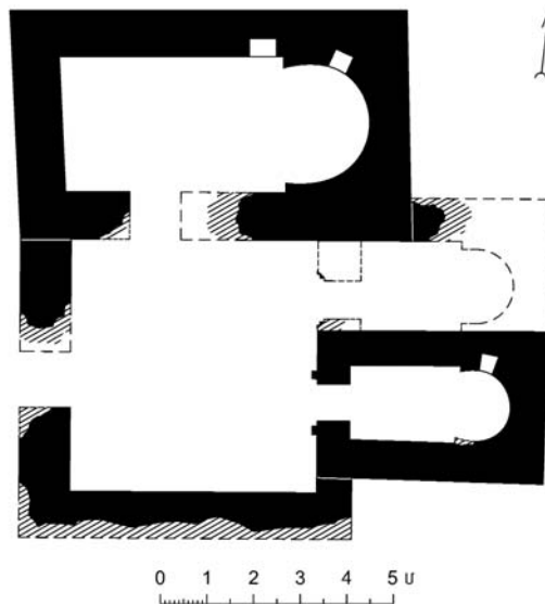
Սր. Մամասի վանքի հատակագիծը (չափ.՝ Ա. Հակոբյանի, 2018 թ.)
