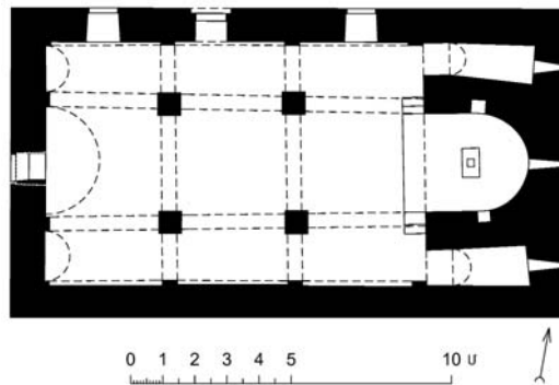
Սր. Խաչ եկեղեցու հատակագիծը (չափ.՝ Ա. Հակոբյանի, 2018 թ.)
