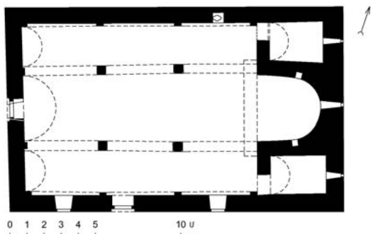
Մր. Խաչ եկեղեցու հատակագիծը (չափ.՝ Ս. Հակոբյանի, 2018 թ.)
