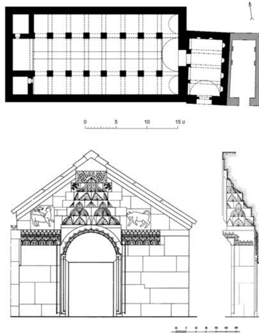
Օրբելյանների իջևանատան (հոգետան) հատակագիծը և նախասրահի հարավային ճակատից բացված շքամուտքը (արտատպված՝ Վ. Հարությունյանի «Միջնադարյան Հայաստանի իջևանատներն ու կամուրջները»/Երևան, 1960, էջ 21/և Ը. Ազատյանի «Շքամուտքերը IV-XIV դդ. Հայաստանի մոնումենտալ ճարտարապետության մեջ»/Երևան, 1987/ գրքերից)
