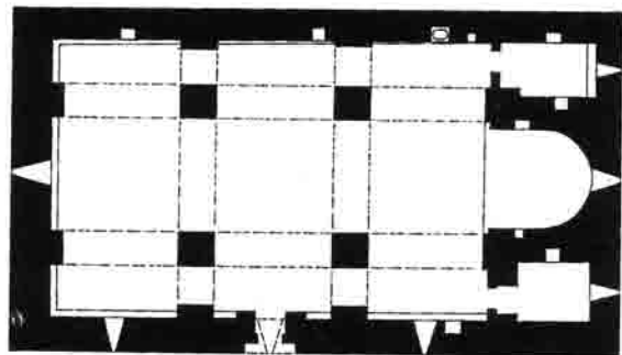
ՅՈՒ. Սր. Մինաս եկեղեցու հասակագիծը
