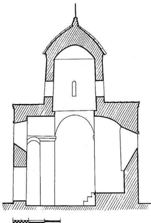
ԳՄՐԵԹԱՎՈՐ ՓՈՔՐ ԵԿԵՂԵՑԻ. արեւմտյան եւ հարավային ճակատները, կտրված դեղի հյուսիս եւ արեւելք (չափագրություն եւ վերակազմություն՝ ճարհ. Սամվել Այվազյանի)
