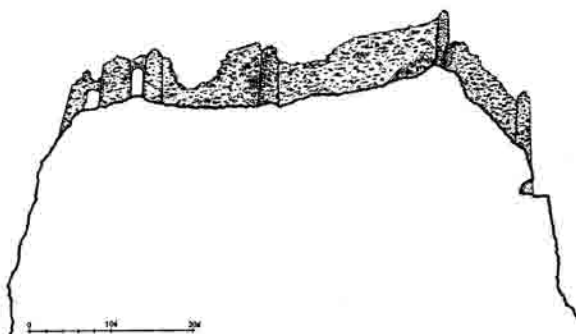
ՀԱՆՂԱԲԵՐԴ, հասակագիծը եւ հյուսիսային ճակատը
