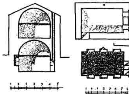
Մելիք Դավթազի աղարանը Քաշաթաղում (չափագրություն՝ ճար. Արսակ Դուլյանի)
