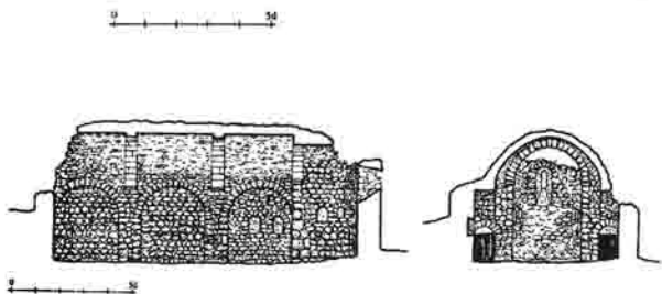
ԵՐԻՑՈՒՇԵՆ. Եկեղեցի գյուղաքեղիում XVII դ., (հասակագիծ, կտրված դեղի հյուսիս եւ արեւել)
