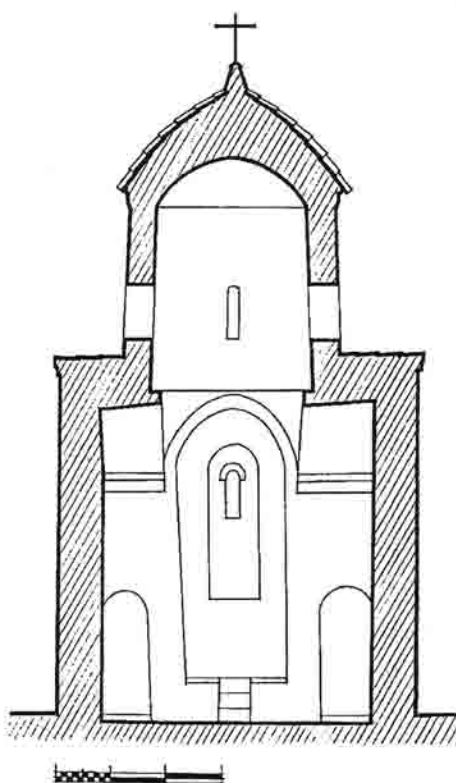
ԳՄՐԵԹԱՎՈՐ ՓՈՔՐ ԵԿԵՂԵՑԻ. արեւմտյան եւ հարավային ճակատները, կտրված դեղի հյուսիս եւ արեւելք (չափագրություն եւ վերակազմություն՝ ճարհ. Սամվել Այվազյանի)
