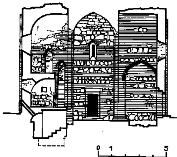
ԳՐԵՄ. Սր. Աստվածածին եկեղեցու կտրվածքը դեպի արևելք և հարավ
