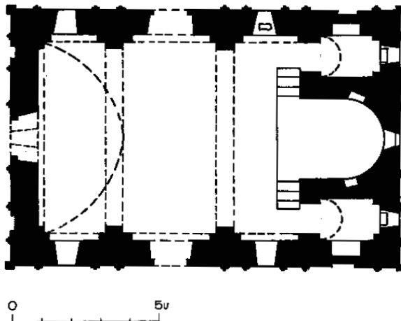
ԹԵԼԱԿ. Սր. Երրորդություն եկեղեցու հատակագիծը
