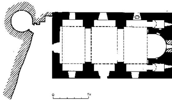
ՎԵԼԻՍՑԻԽԵ. Սր. Աստվածածին եկեղեցու հատակագիծը
