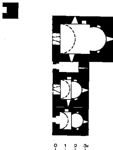
ԳՐԵՄ. Եկեղեցին արևմուտքից և արևելքից, ներքին տեսքը դեպի արևմուտք և հարավից կից ավանդատուն-սրահի արևելյան ճակատում (արտաքուստ) ագուցված խաչքարերից մեկը ԳՐԵՄ. Եկեղեցու, մատուռ-զանգակատան, մատուռի և որմնափակ խաչքարի հատակագիծը
