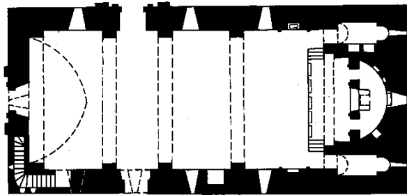
ԹԵԼԱՎ. Չվեղավալանի Սր. Գեորգ եկեղեցու հատակագիծը
