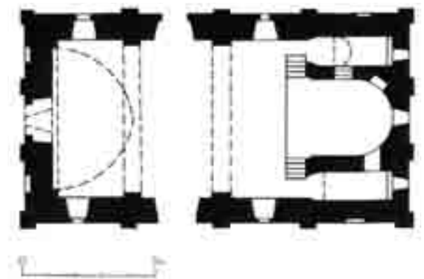
ՈՐԻՆԱԹՈՒՐԱՆ. Սր. Սարգիս եկեղեցու հատակագիծը
