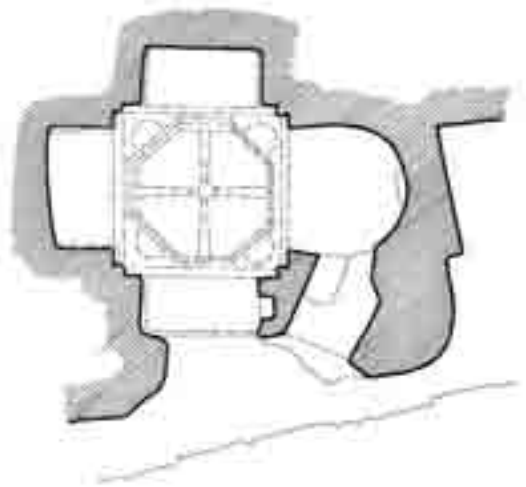
ՍԱԲԵՐԵԲԻ. պայմանական № 7 եկեղեցու հատակագիծը
