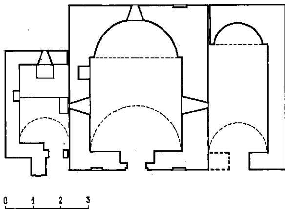
ԳՐԵՄ. եկեղեցու (№10) հատակագիծը. չափագրությունը՝ Մ. Դասրաթյանի
