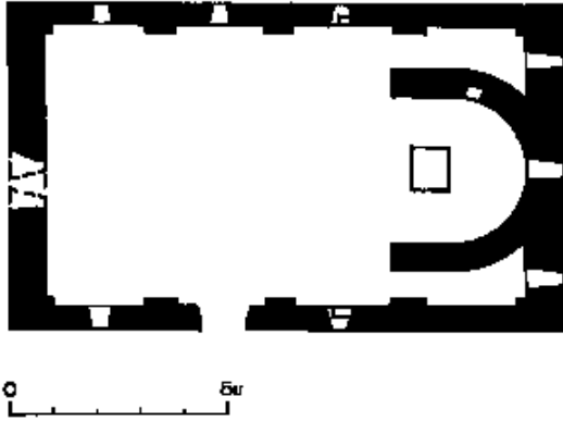
ՄՍՏԱՆ. Սր. Աստվածածին եկեղեցու հատակագիծը
