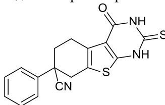
Соединение 10: 4-Оксо-7-фенил-2-тиоксо-1,2,3,4,5,6,7,8-октагидробензо[4,5]тиено[2,3- d ] пиримидин-7-карбонитрил:
