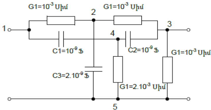
Նկ. 2.ա -Կրկնակի կամրջակային սխեմա
