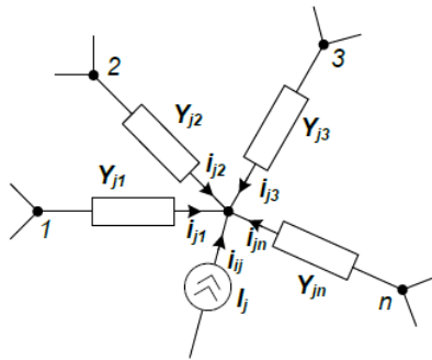
Նկ. 1. n -հանգույցով պասիվ սխեմայի տեղամաս:
