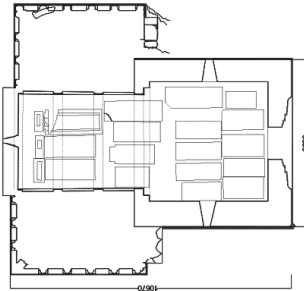
Նկ. 1. Վանական համալիրի հատակագիծը (չափ. Հ. Խալիֆախյանի)
