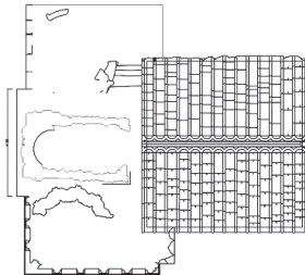
Նկ. 3. Զամարյանների դամբարանի չափագրություններ (Հուշարձաններ վերականգնող հարտարապետների հայկական ասոցիացիա)
