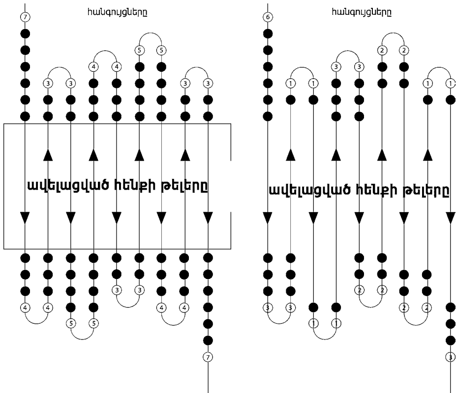
Նկ. 5 ա, բ. Ուղղահայաց թելերի՝ հիմնաթելի անցկացման տեխնիկական գծագիր:
