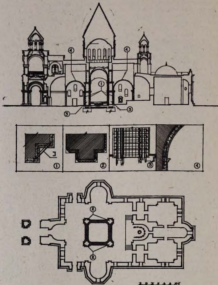
Քժ. 3. Մայր տաճարի զմբեթակիր մույթերի և կամարների ամրացման նախագիծ:
