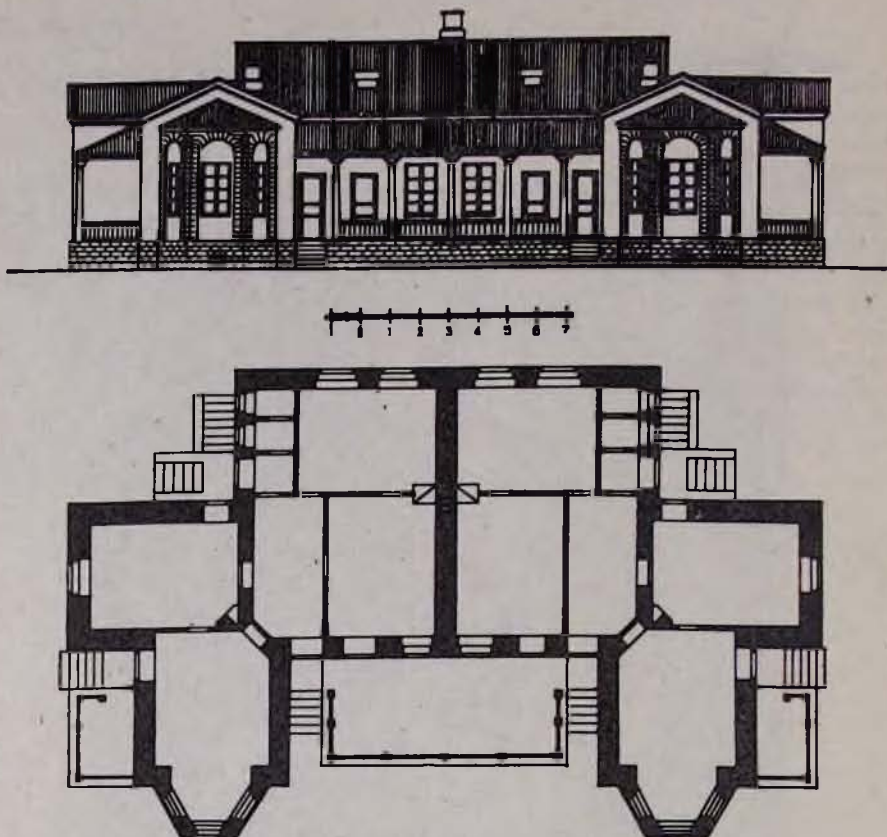
Նկ. 2. Լուվաշեն. կցաշար միահարկ բնակելի տան տիպ. հատակագիծ և ճակատ:
