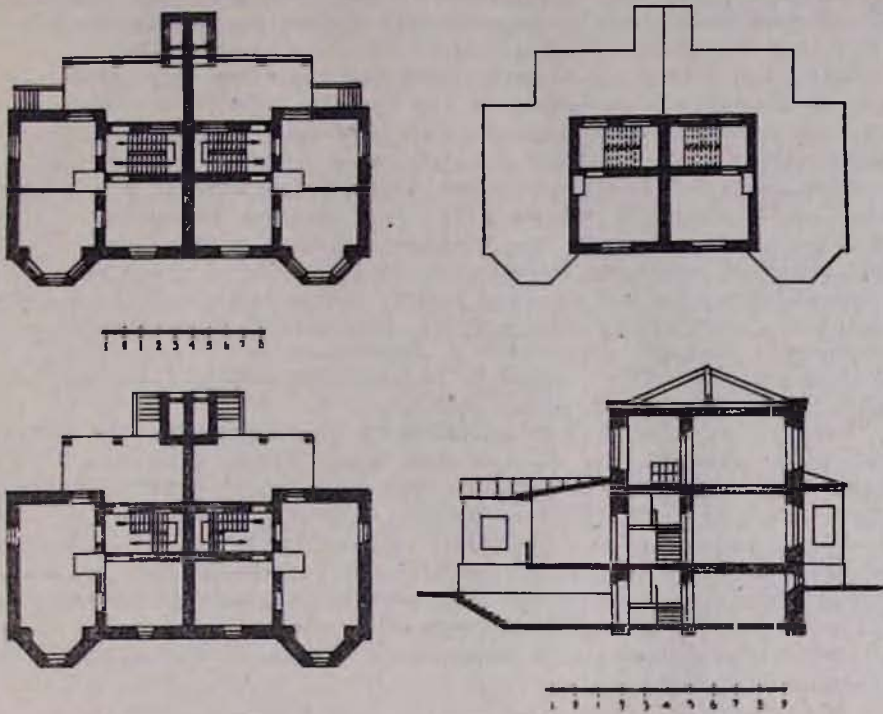
Նկ. 7. Նուրարաշեն. կցաշար երկհարկ բնակելի տան տիպ. հատակագծեր և կտրվածք:
