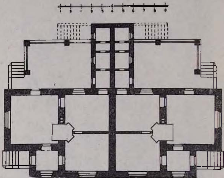
Նկ. 6. Նուբարաշեն. կցաշար միահարկ բնակելի տան տիպ:
