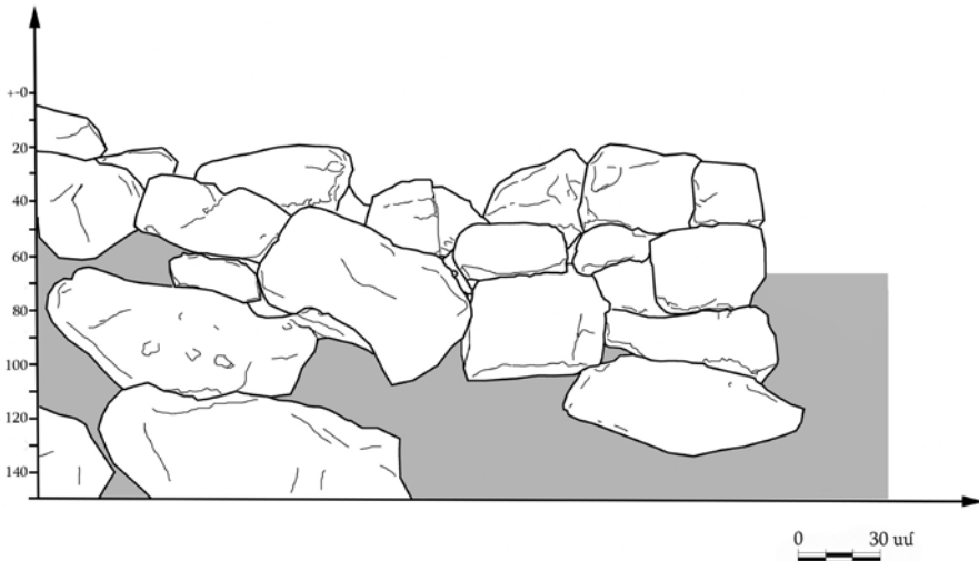
Նկ. 8. Անտառուս 1 դղյակի պարաշարը (չափագրությունը՝ Հ. Դանիելյանի)
