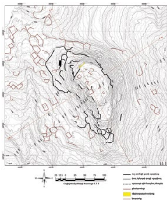
Նկ. 5. Բազմադրյուր 1 ամրացված քնակալեղիի տեղագրական հանույթ (հանույթը՝ Հ. Դանիելյանի)
