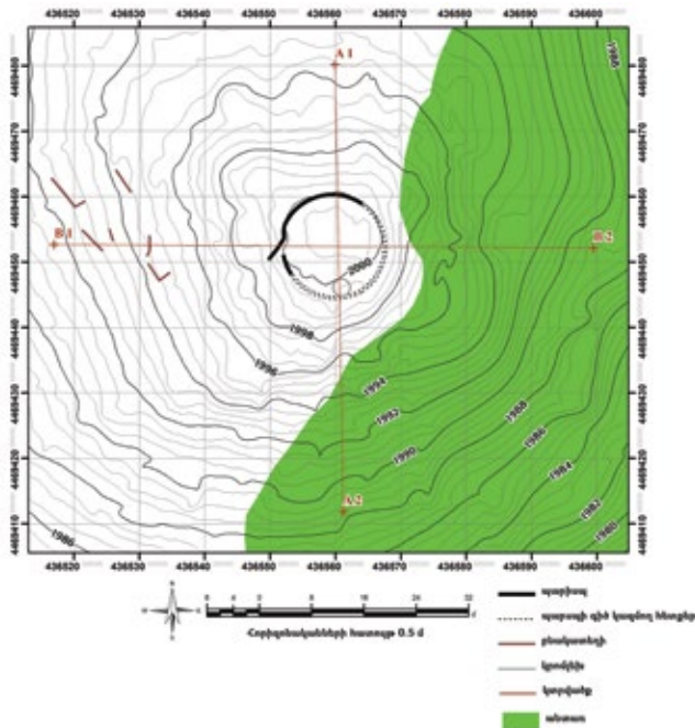
Նկ. 2. Բյուրական 1 ամրոցի տեղագրական հանույթը (հանույթը՝ Հ. Դանիելյանի)
