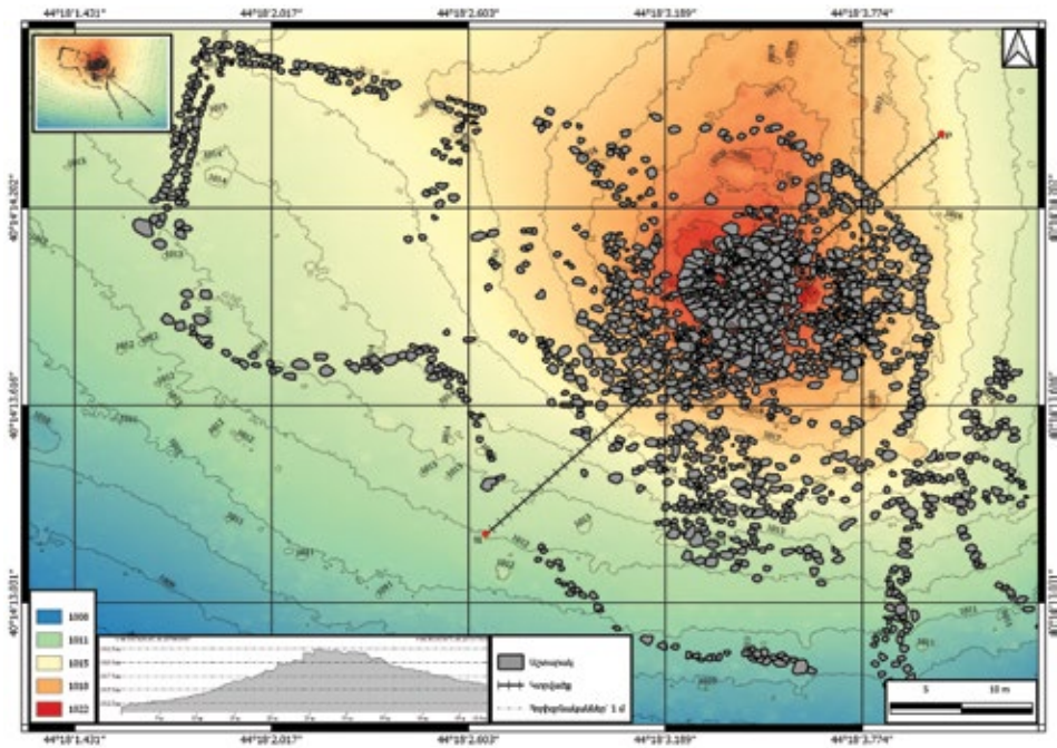
Նկ. 4. Արղար Դալիթի հանույթն ու հատակագիծը (կազմող՝ Լ. Մկրտչյան)
