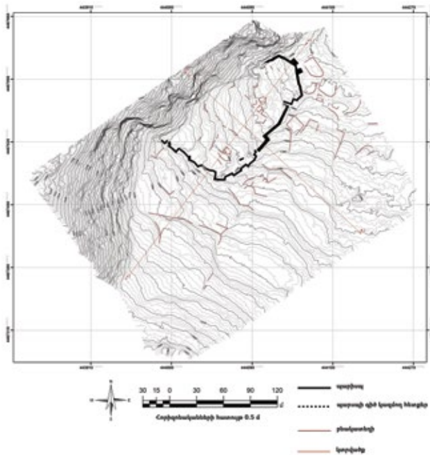
Նկ. 4. Հազարավան 1 ամրացված բնակավտեղիի տեղագրական հանույթ (հանույթը՝ Հ. Դանիելյանի)
