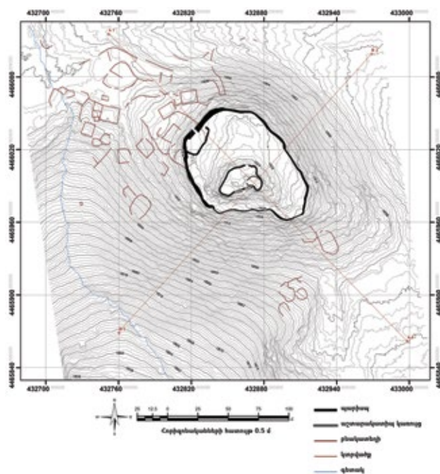
Նկ. 6. Ավան 1 ամրացված բնակատեղիի տեղագրական հանույթ (հանույթը՝ Հ. Դանիելյանի)
