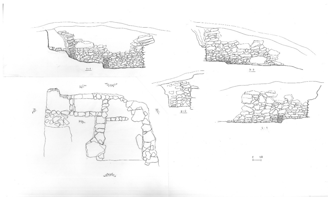
Նկ. 7 Ենթադրյալ դամբարանային համալիրը
