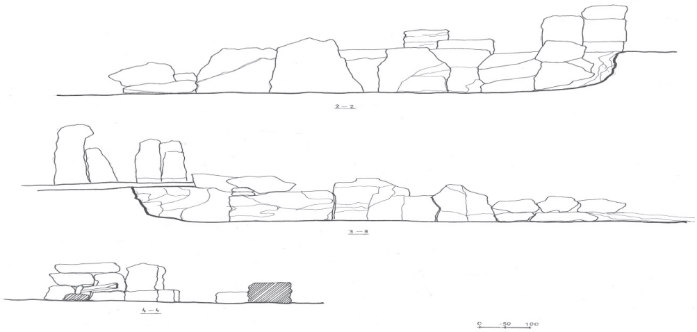
նկ. 4 Տաճարին կից ժայռափոր սենյակի կտրվածքը
