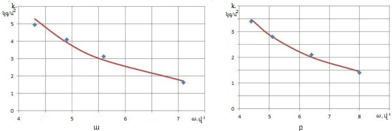
Նկ. 3. 15 մմ-ից մեծ կոշտերի քանակի կախվածությունը ռոտորային կոշտամանրիչի անկյունային արագությունից. \omega - թեթև կավավազային հողատիպ, p - ծանր կավավազային հողատիպ:
