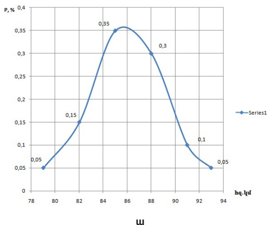
Սկ. 1. Սուպորտի միացի ուղղորդ մատի (ա) և միջին ռեսուրսի (բ) բաշխման տեսական կորերը:
