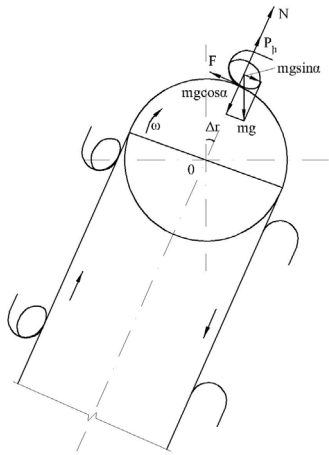
Նկ. 3. Պալարների անկման \alpha_{\min} և \alpha_{\max} անկյունների համապատասխան հետազոծերի սխեման:
