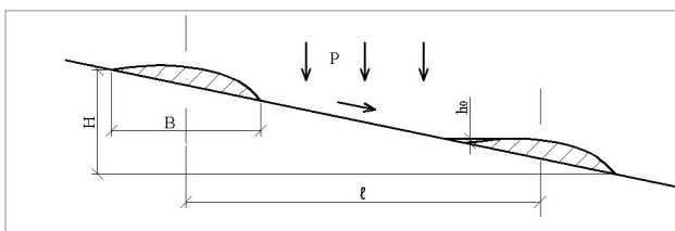
Նկ. 1. Կատարավոր դարավանդի սխեման:
