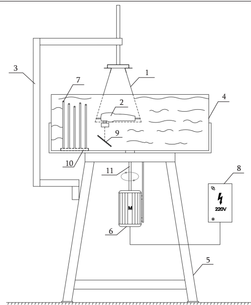
Նկ. 1. Ջրային միջավայրում բույսերի ցողունների վիբրացիոն կտրման փորձարարական կայանի ընդհանուր սխեման: 1 - իրան, 2 - էլեկտրամագնիսական վիբրատոր, 3 - մետաղյա ձող, 4 - ջրով լցված տարա, 5 - սեղան, 6 - շարժիչ, 7 - եղեգնի ցողուն, 8 - կերպափոխիչ, 9 - վիբրացիոն դանակի սայր, 10 - մետաղյա ափսե, 11 - 30 սմ երկարությամբ ձող (կազմվել է հեղինակի կողմից):
