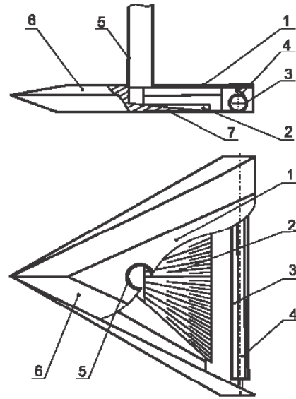
Նկ. 1. Շաղացանի սերմադիչ խոփիկի կառուցվածքային սխեման:
