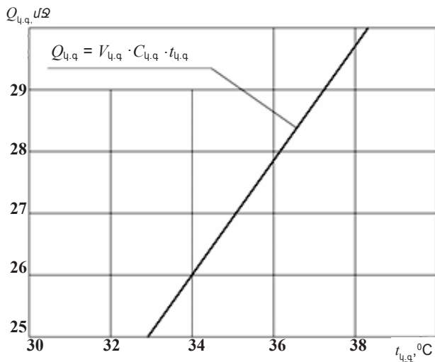
Նկ. 2. Կենսագազի հետ մեթանտենկից դուրս եկած ջերմության քանակի փոփոխությունն ըստ խմորվող սուբստրատի ջերմաստիճանի (կազմվել է հեղինակների կողմից):
