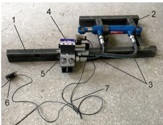
Նկ. 2. Բանող օրգանների էլեկտրամեխանիկական եղանակով կառավարման հանգույցի փորձանմուշը և փորձարկման ստենդը. 1 - Կառավարման, 2 - Կառավարման փորձարկման ստենդը, 3 - Բարձր ճնշման ծկախողովակներ, 4 - Էլեկտրամագնիսական հիդրոբաշխիչ, 5 - Սալիկ, 6 - Վերջնային անջատիչ, 7 - Հաղորդակար:
