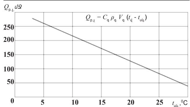
Նկ. 1. Գոմաղբի օրվա բաժնաչափի շերմաստիճանը մինչև +34^\circ\text{C} հասցնելու շերմության ծախսի փոփոխությունն ըստ մեթանտենկ մատուցվող գոմաղբի շերմաստիճանի (կազմվել է հեղինակների կողմից):
