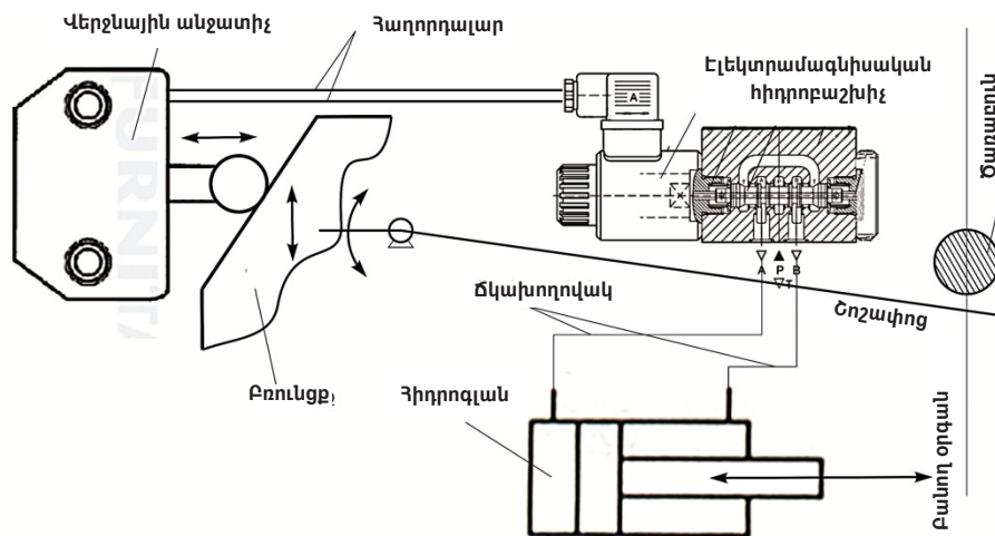
Նկ. 1. Բանող օրգանների էլեկտրամեխանիկական եղանակով կառավարման սխեման (կազմվել է հեղինակների կողմից):
