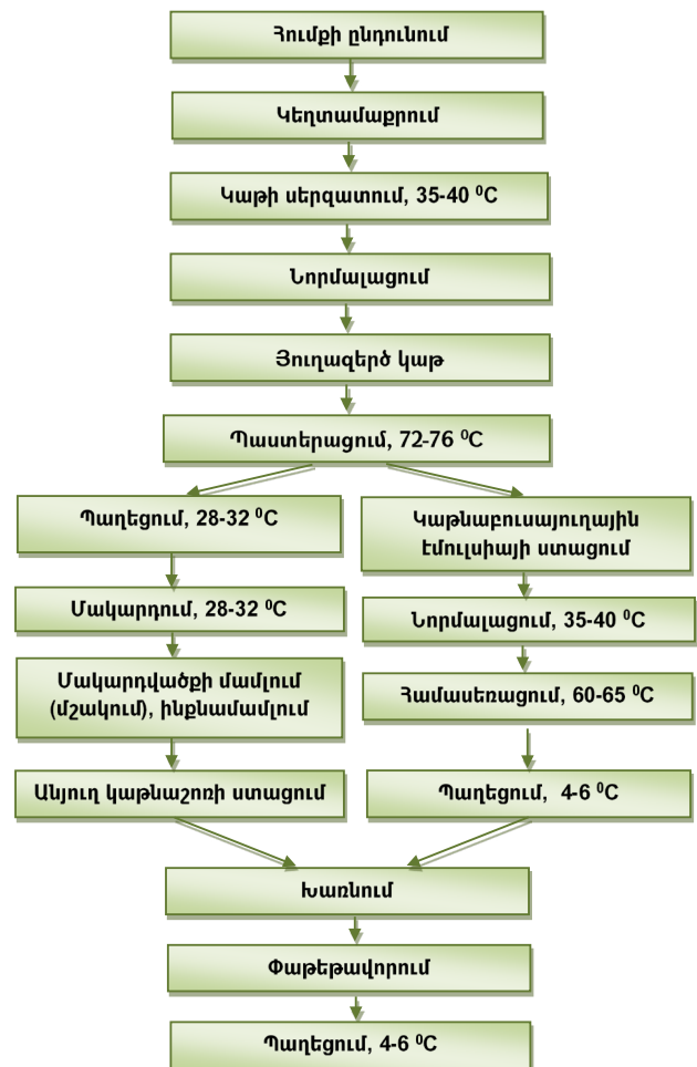
Նկ. 6. Զիրապտղի յուղով հարստացված կաթնաշոռային զանգվածի արտադրության տեխնոլոգիական սխեման (կազմվել է հեղինակների կողմից):
