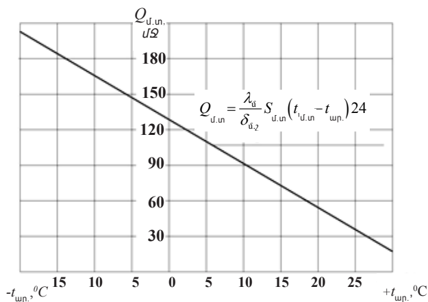
Նկ. 3. Մեթանտենկի մակերեսի մեկուսիչ շերտով ջերմության կորուստների փոփոխությունն ըստ արտաքին միջավայրի օդի ջերմաստիճանի (կազմվել է հեղինակների կողմից):
