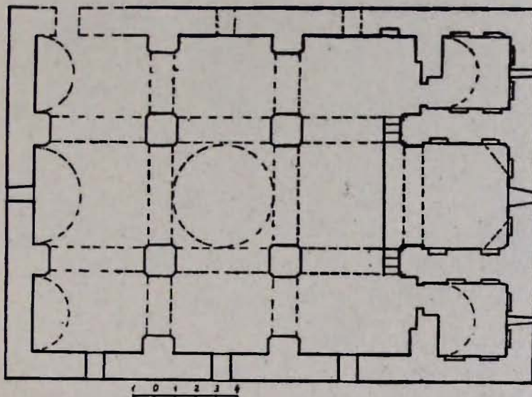
Նկ. 6. Ագուլիսի ս. Հովհաննես-Մկրտիչ եկեղեցու հատակագիծը (չափադրությունը Ա. Ավագյանի):
