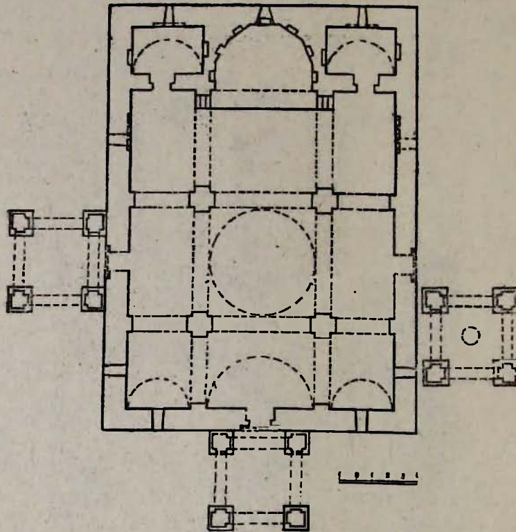
Նկ. 2. Ագուլիսի ս. Թովմա տաճարի գլխավոր հատակագիծը (չափագրությունը Ա. Այվազյանի):
