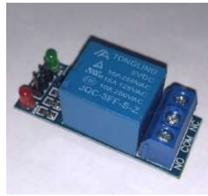
Նկ. 5. Ռելե:
