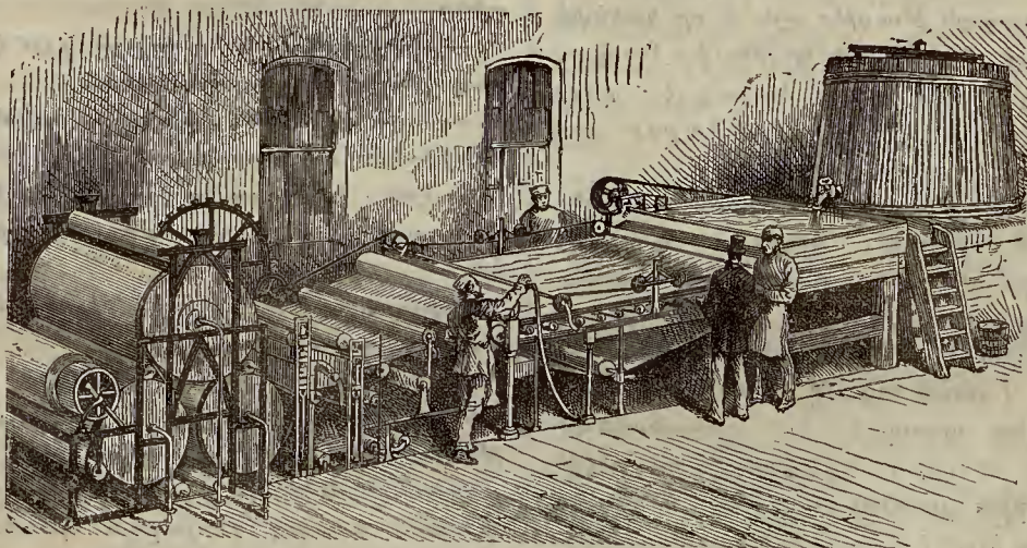
Թուղթ շինող շոգեշարժ մեքենայ
