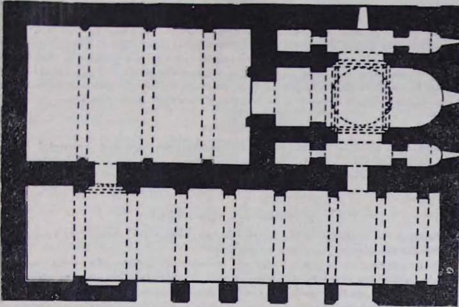
Նկ. 1. Վահանավանք: Կր. Լուսավորիչ եկեղեցու, զավթի և սյունասրահի մոտավոր վերտ-կադմական հատակադիծ: Ճարտարապետներ Ա. Մեսլյան և Լ. Մելիքյան
