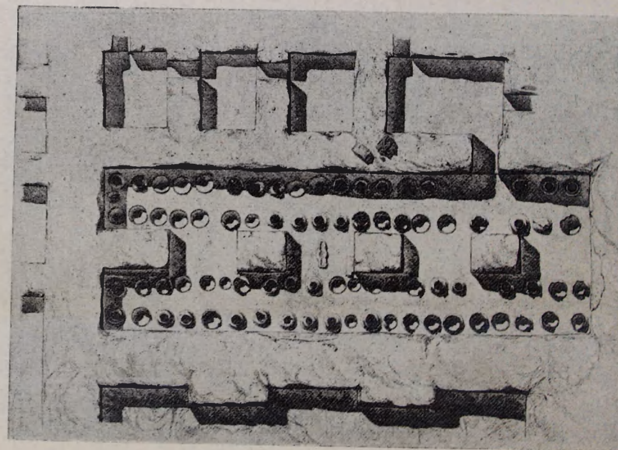
Табл. 6. План кладовой № 25 (обмеры К. Л. Оганесяна).
