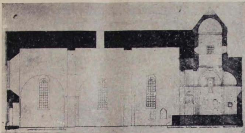
Նկ. № 5. Կաթողիկոս եկեղեցու կտրվածքը հետադարյան հավելվածների հետ միասին: Չափագրություն Տարագրոսի
