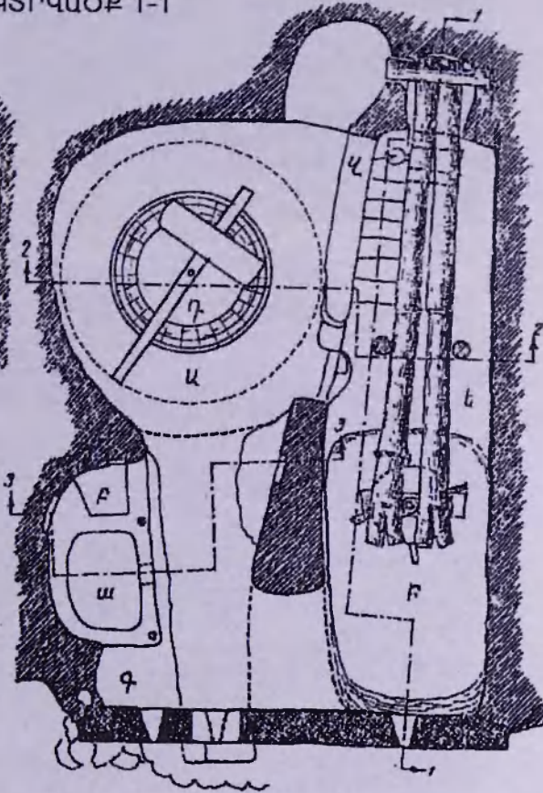
ԿՏՐՎԱԾՔ 1-1
