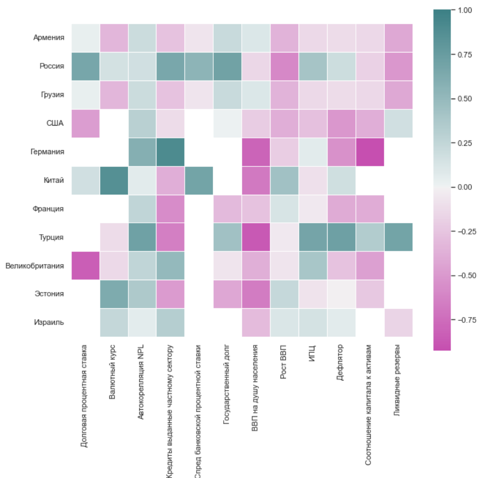
Рис. 1. Тепловая карта, показывающая корреляцию показателей с NPL для разных стран 1
