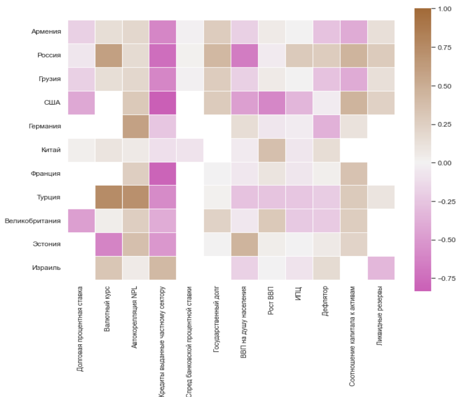
Рис. 2. Тепловая карта, показывающая корреляцию показателей с NPL для разных стран 1
