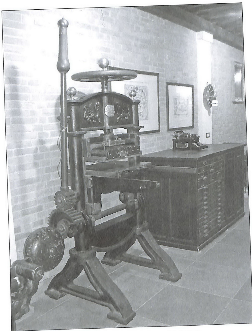
ՏՊԱԳՐԱԿԱՆ ՈՍԿԵՆԱԽՇՈՂ, ՄԱՄԼԻԶ
