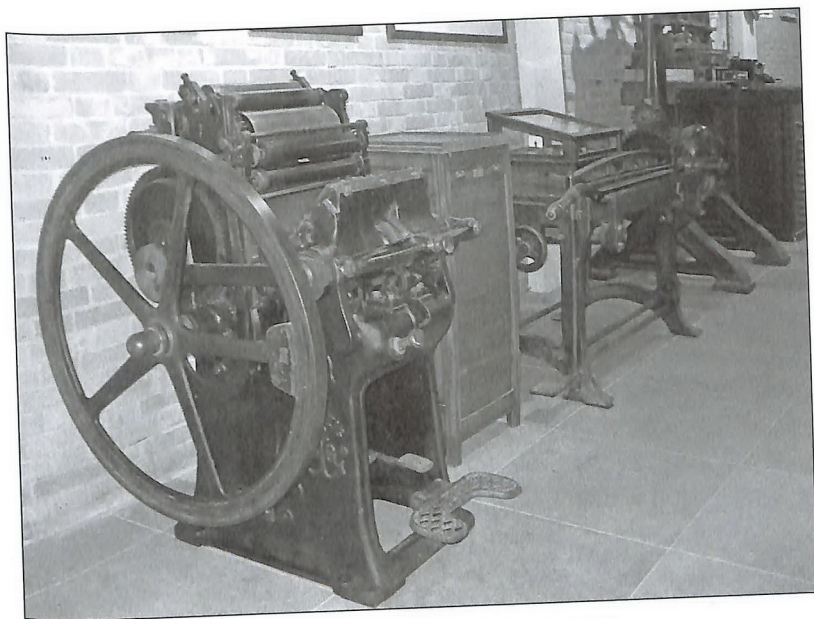
ՏՊԱԳՐԱԿԱՆ ՄԱՄԼԻԶ ՈՏՆԱԿՈՎ
