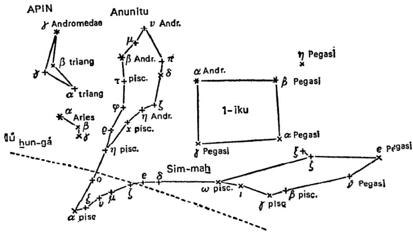
Նկ. 8. Հինմիջագետքեան աստղային ֆարսէզի հատուածը՝ երկնային Արտի եւ Երկնքի տիրումի համաստեղութիւններով: Քարտէզի ստորին մասով անցնող ընդհատ գիծը խաւարածիրն է (ֆարսէզը վերցուած է Վան-Ռե-Վարդէնի գրքից):
